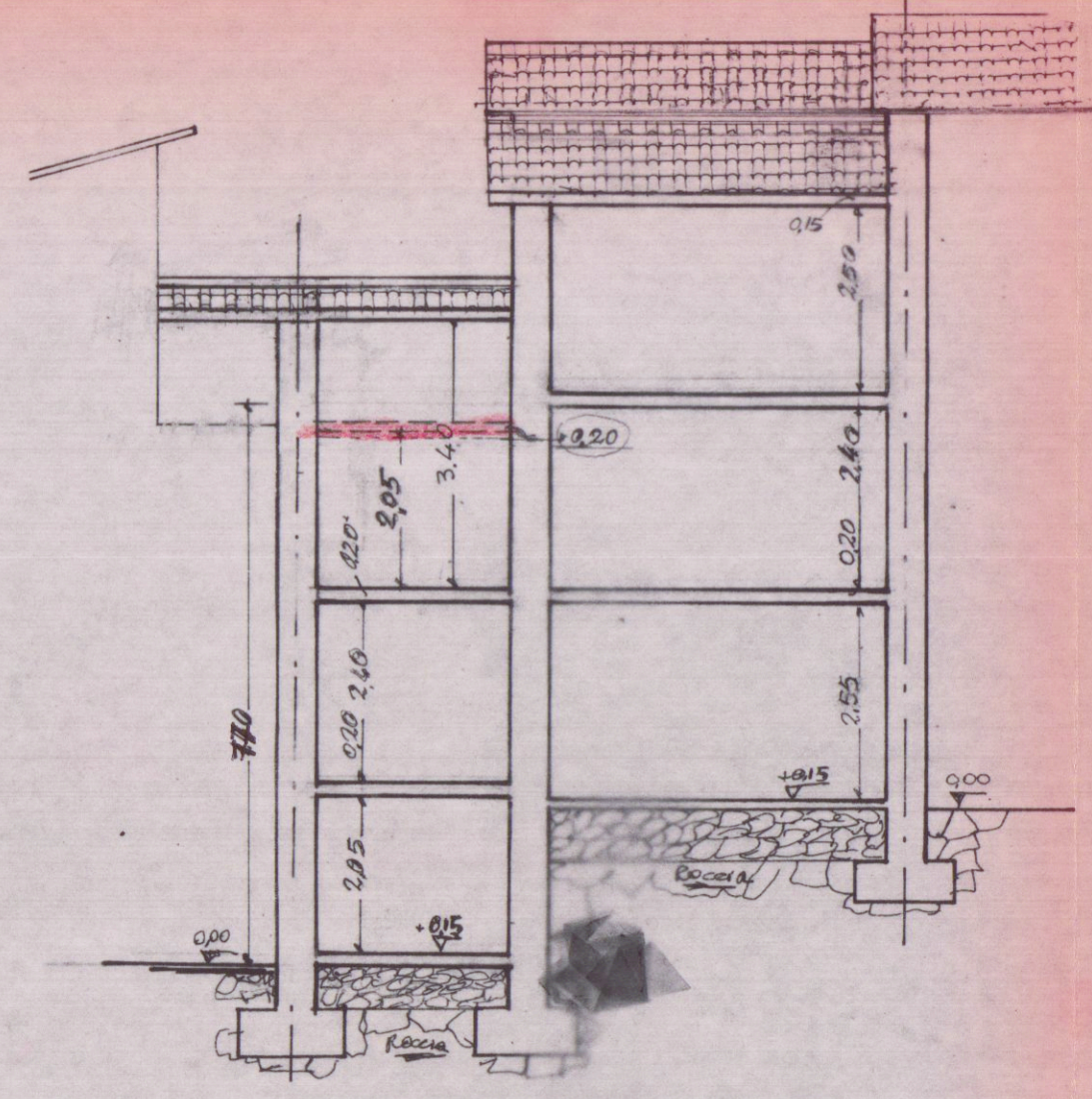
Sezione A-A
