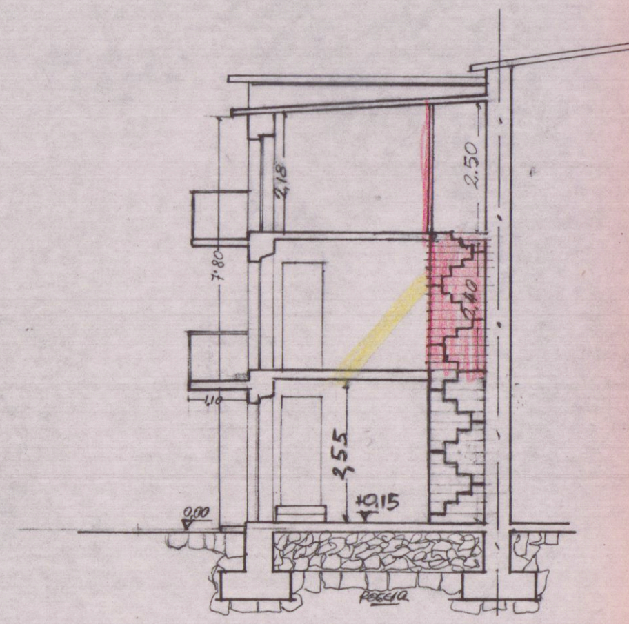
Sezione B-B
