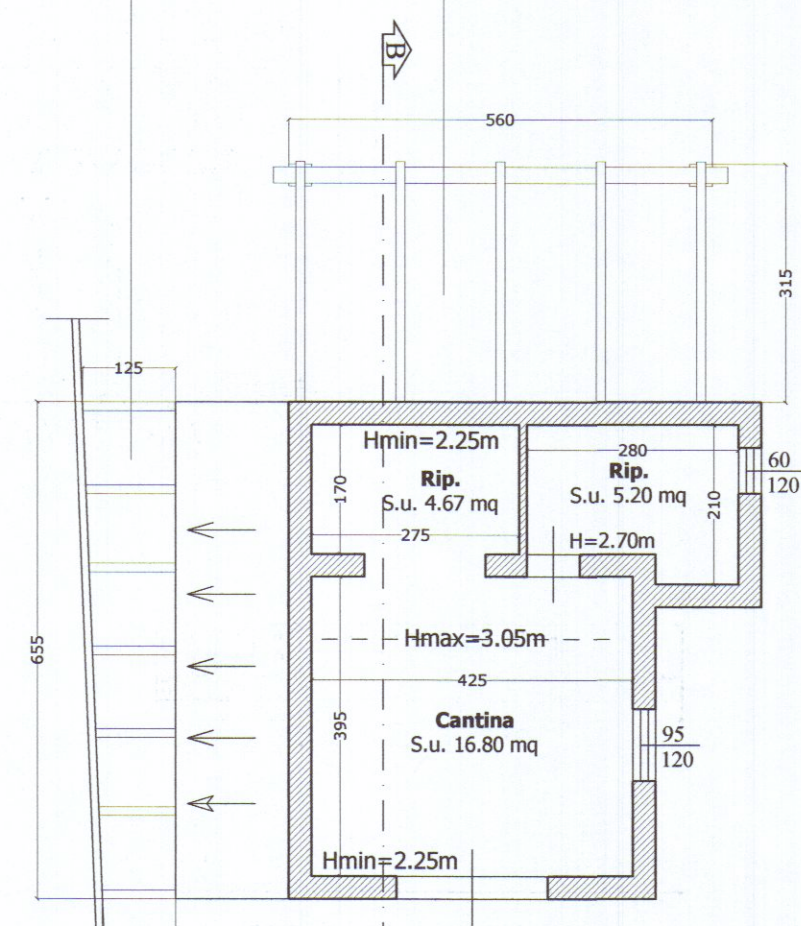
PIANO TERRA CASETTA
