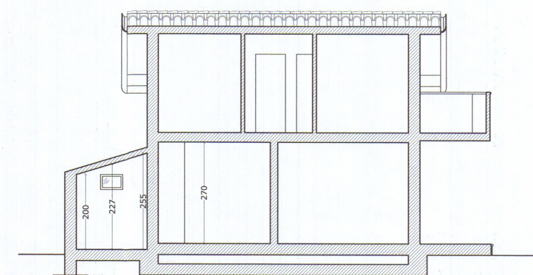
SEZIONE A-A
