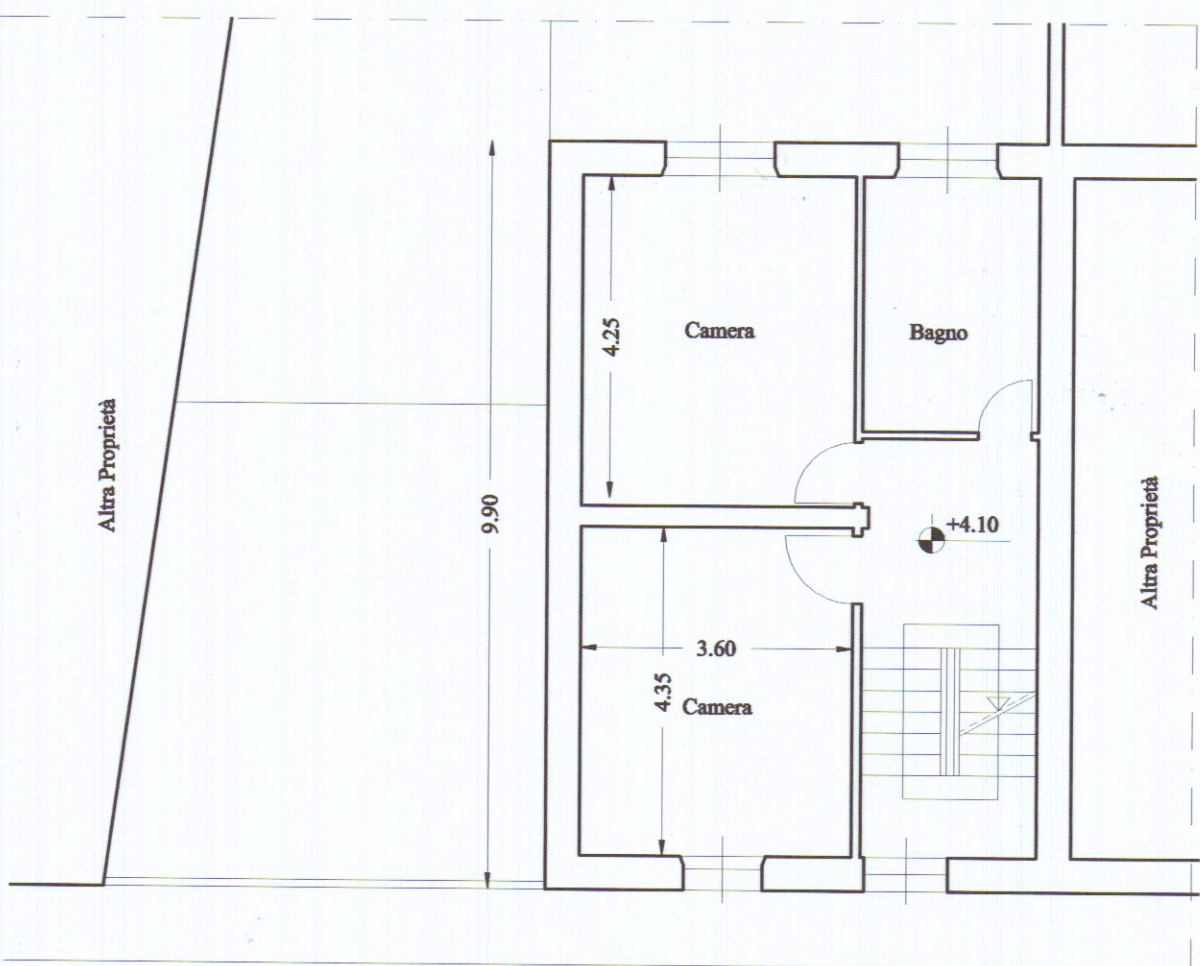
PIANTA PIANO PRIMO DI PROGETTO
