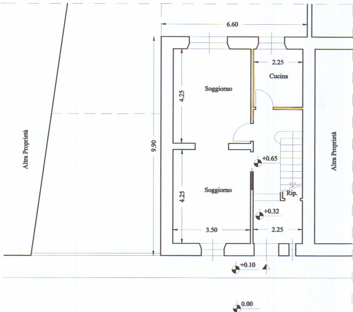
PIANTA PIANO TERRA DI PROGETTO
