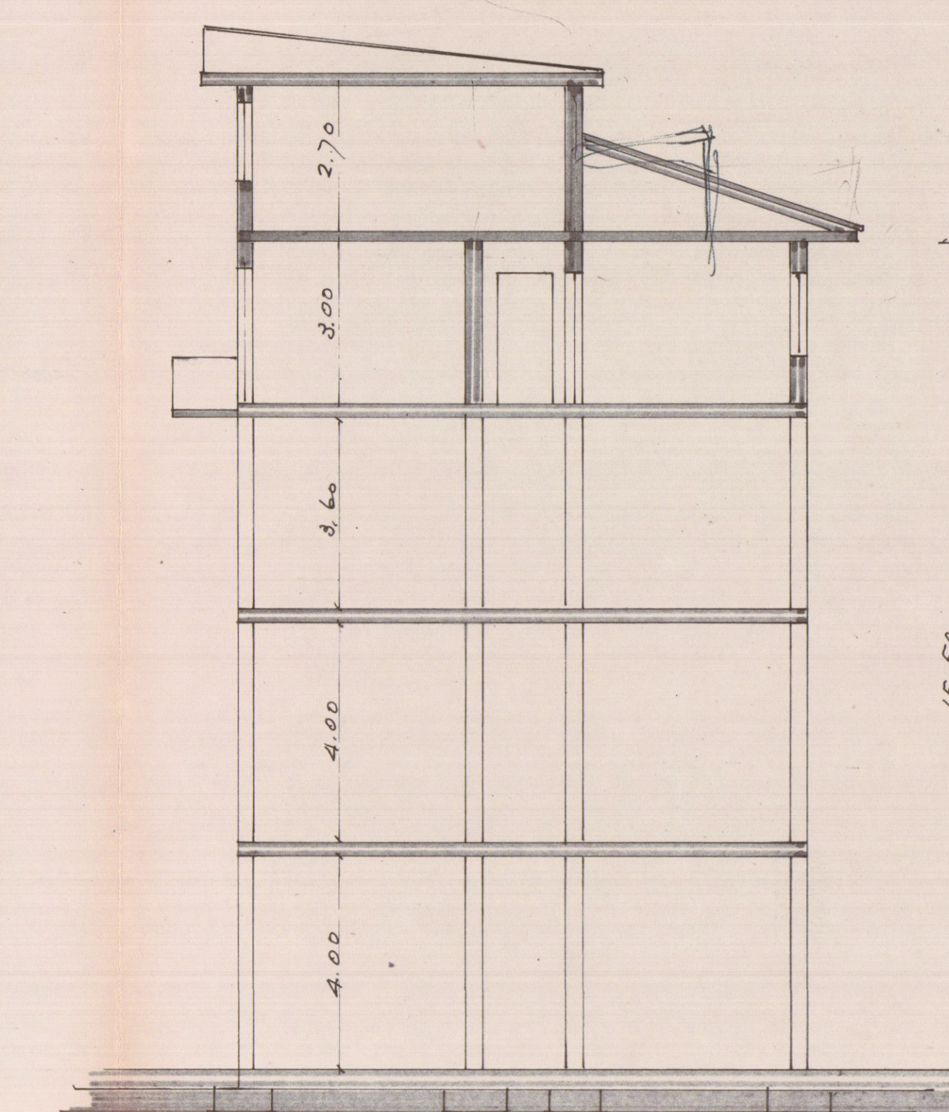
Sezione A-B
