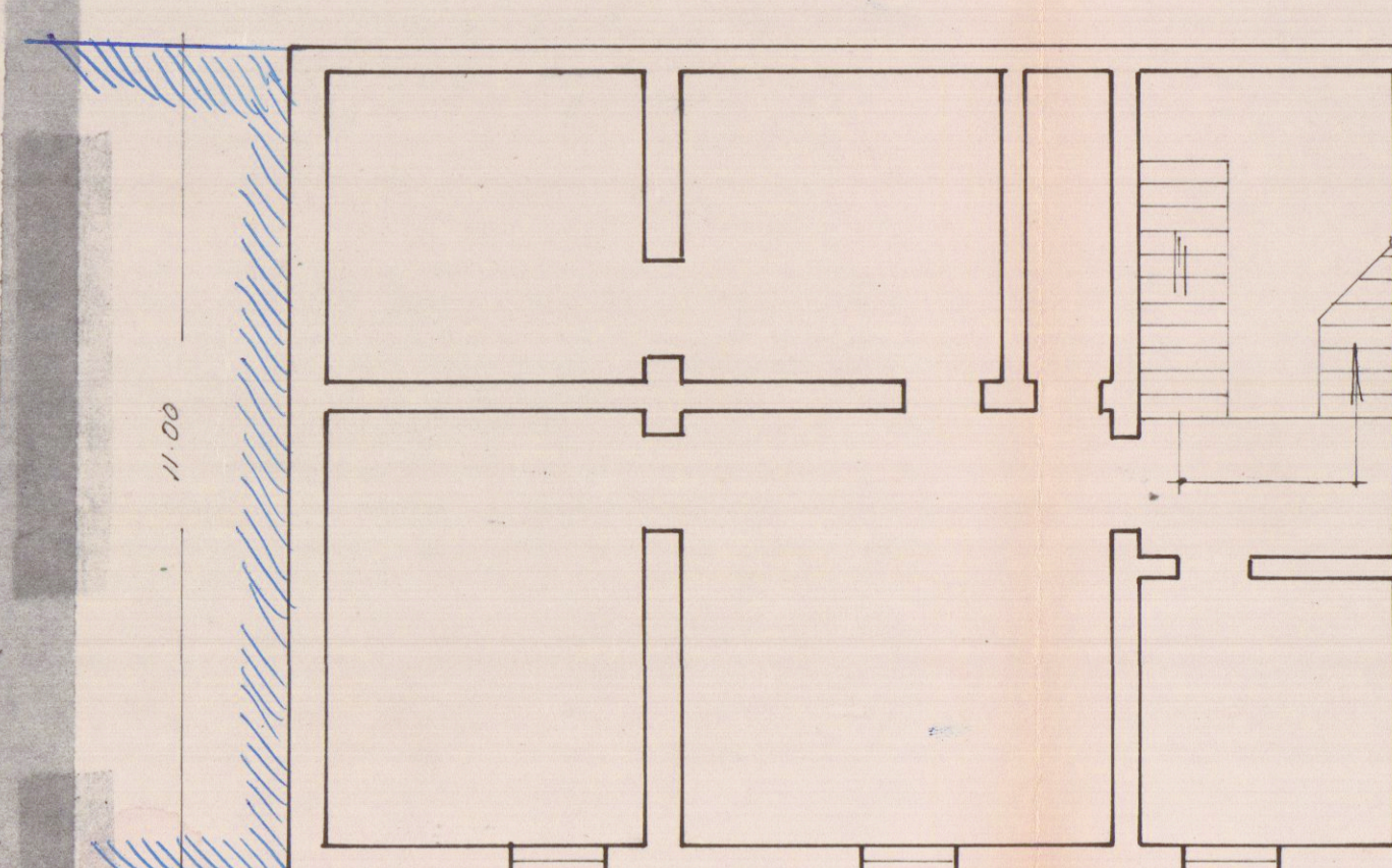
pianta esistente via Lunense
