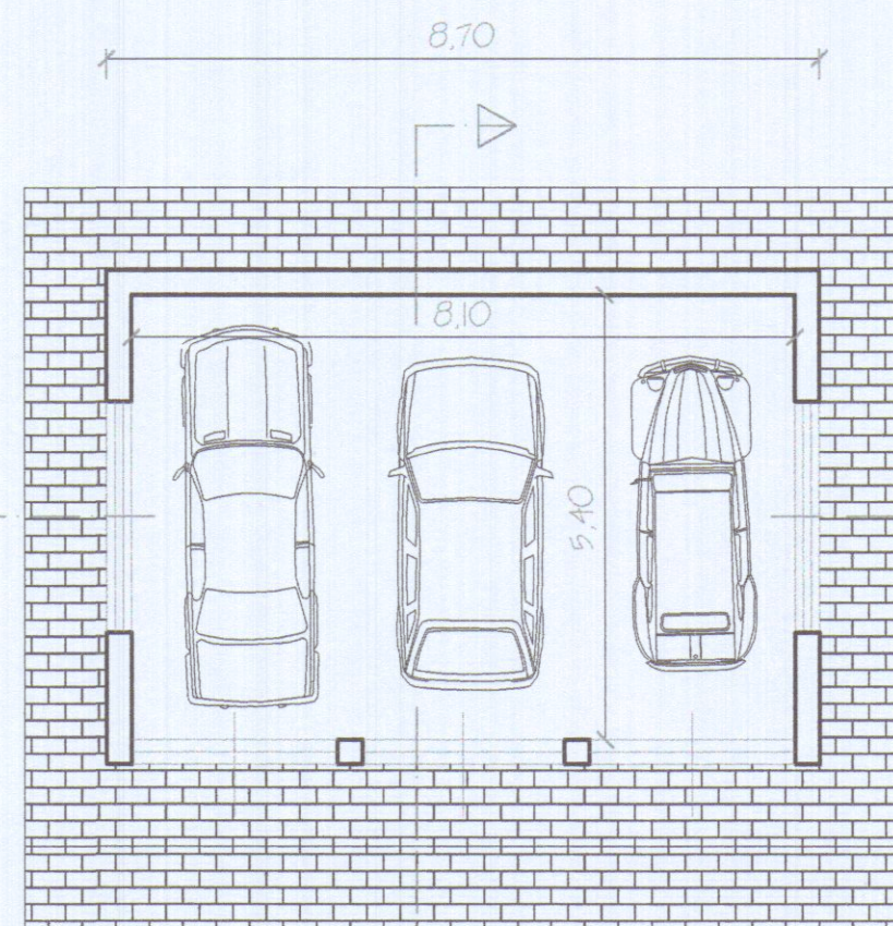
PIANTA
