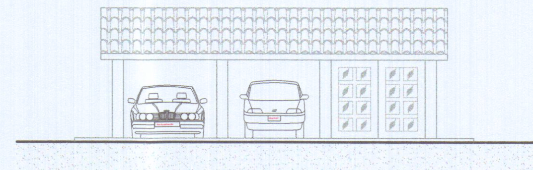
PROSPETTO SUD
