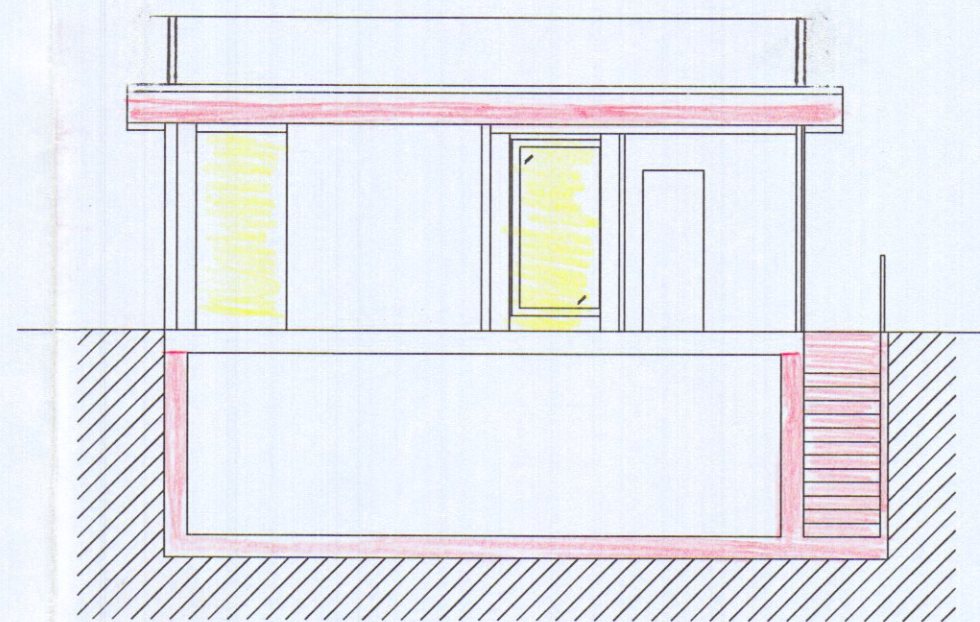
Sezione YY''
