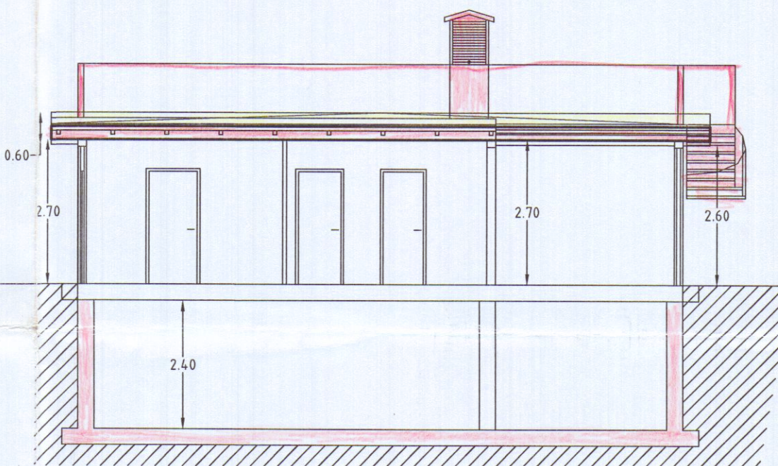
Sezione XX'
