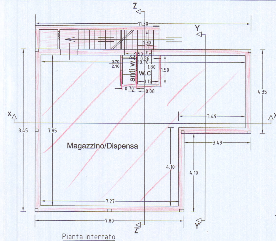
Pianta Interrato
