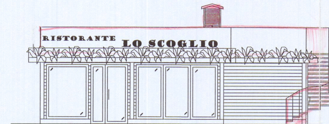
Prospetto Sud-Est
