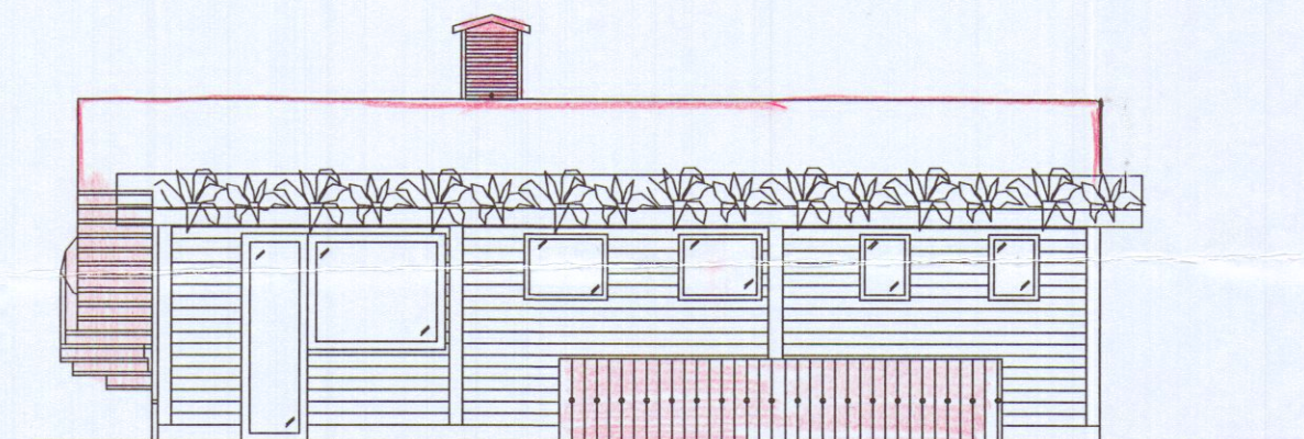
Prospetto Nord-Ovest
