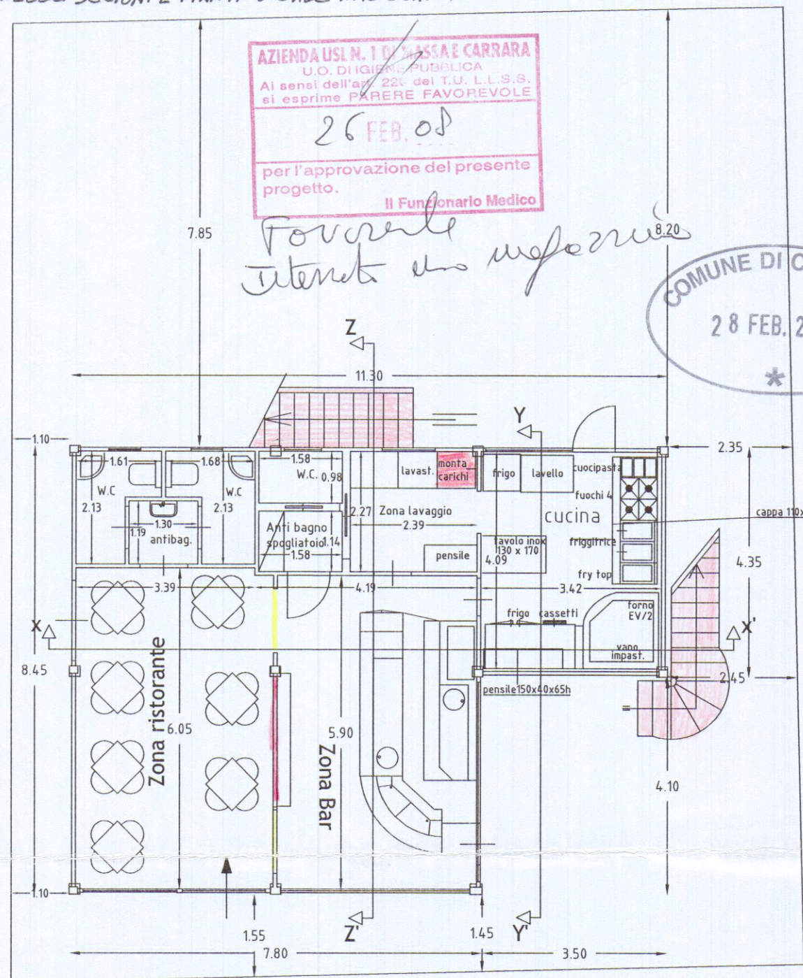
Pianta
