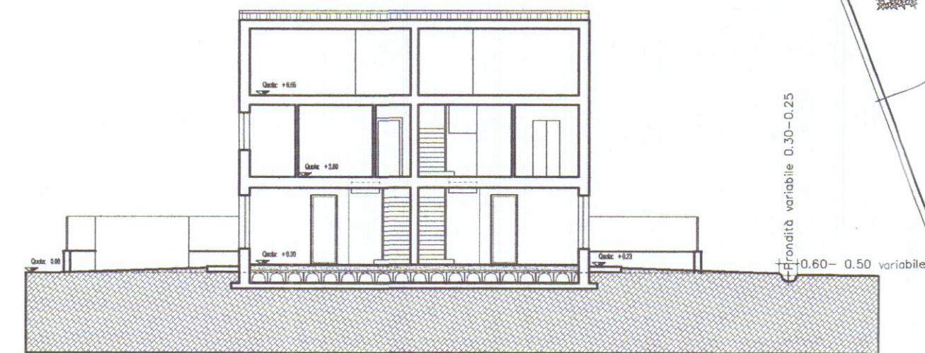
Sezione B-B
