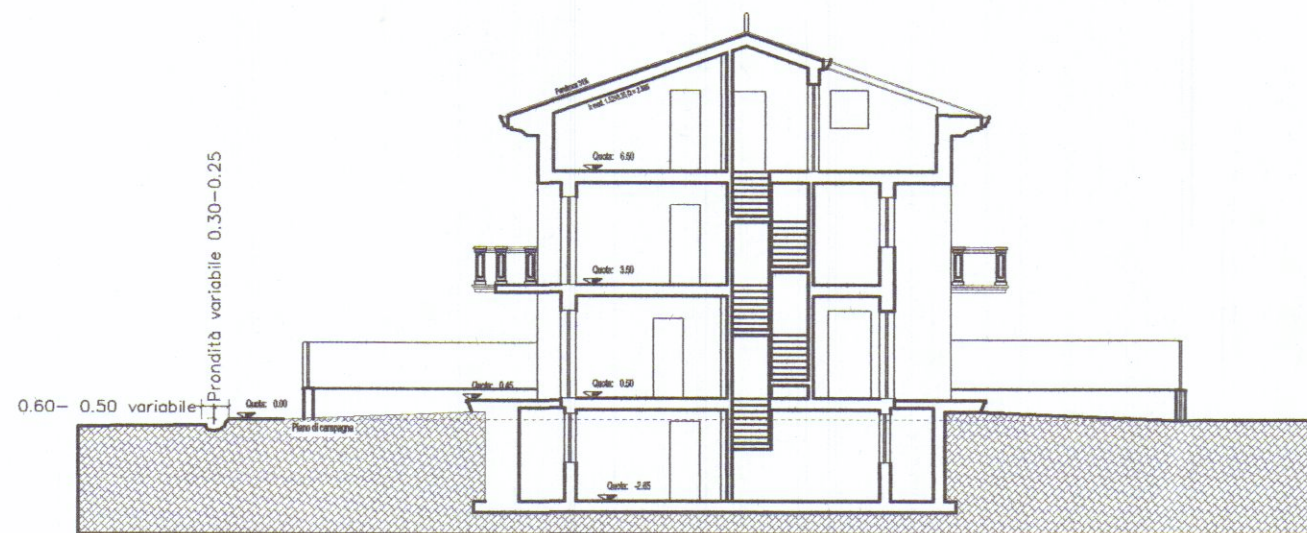
Sezione A-A
