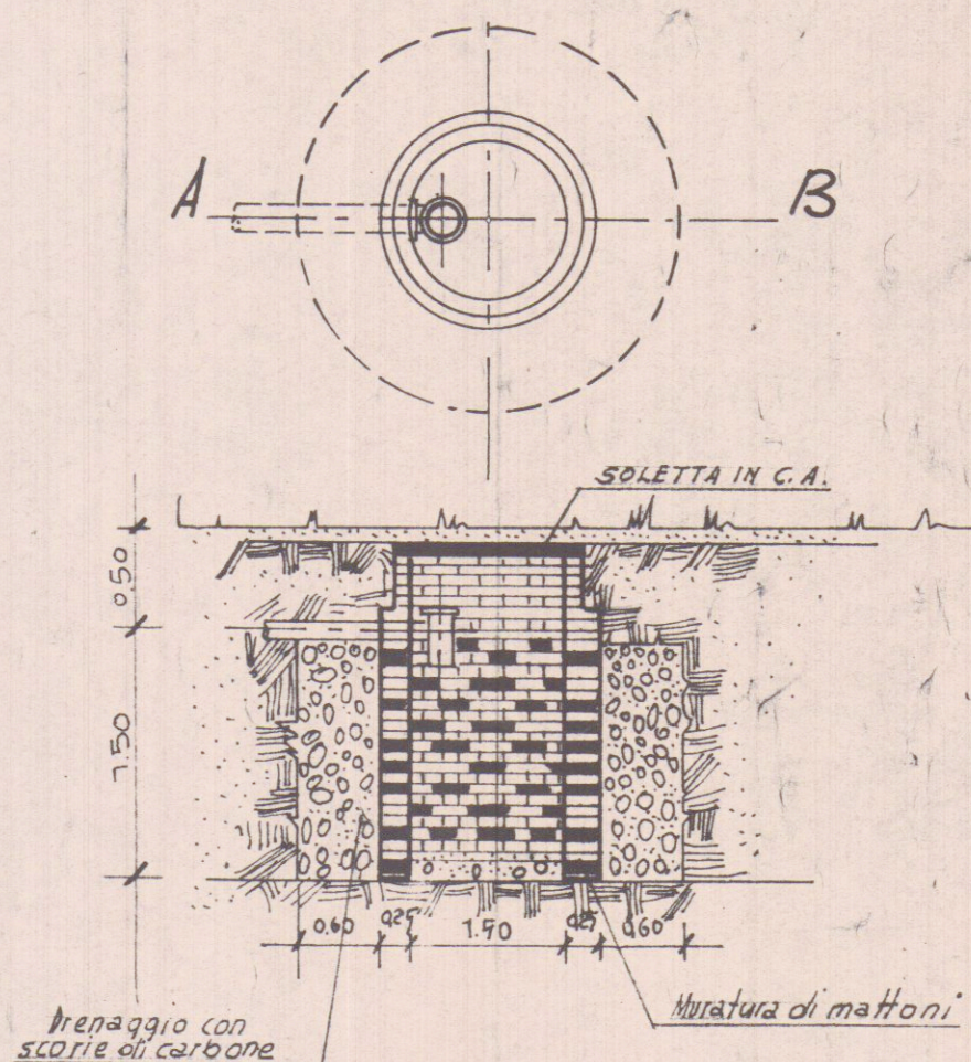
SEZIONE A.B
