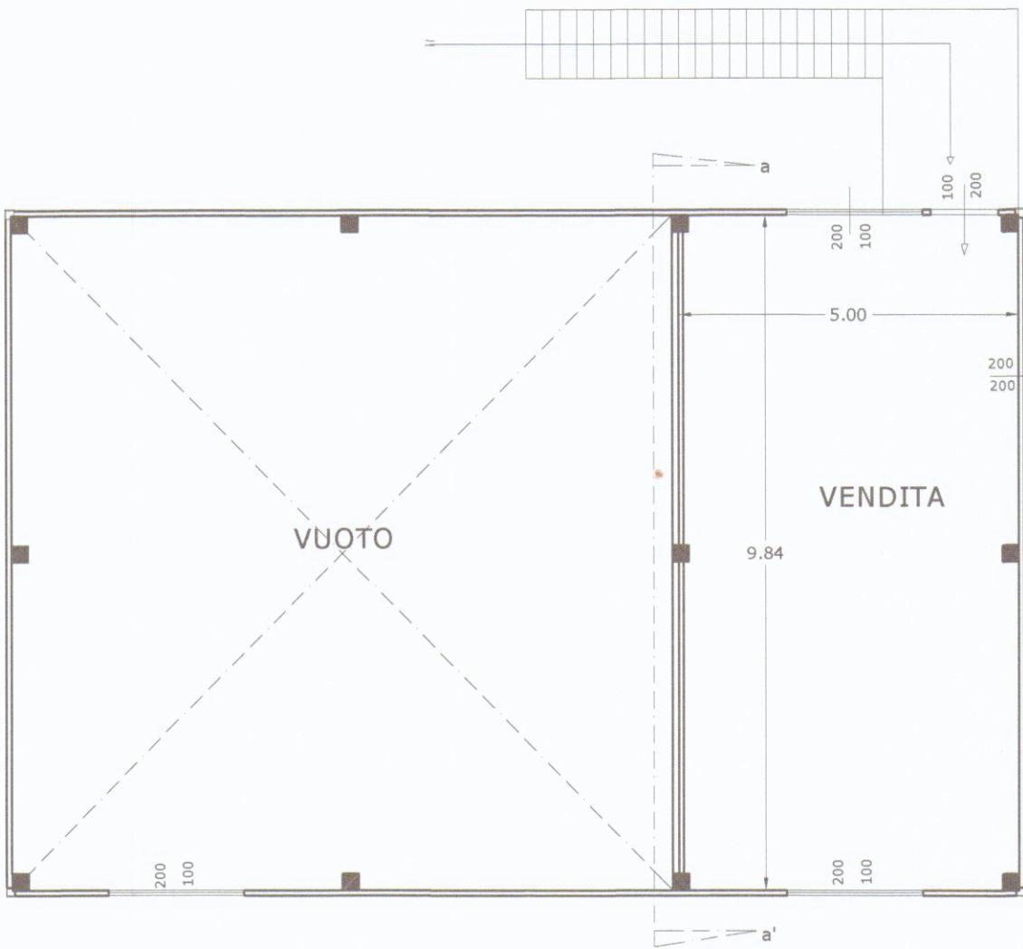
PIANTA PRIMO
