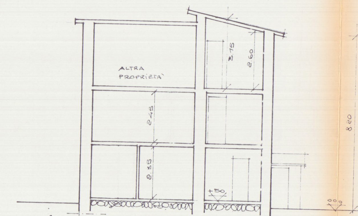
SEZIONE A-A'
