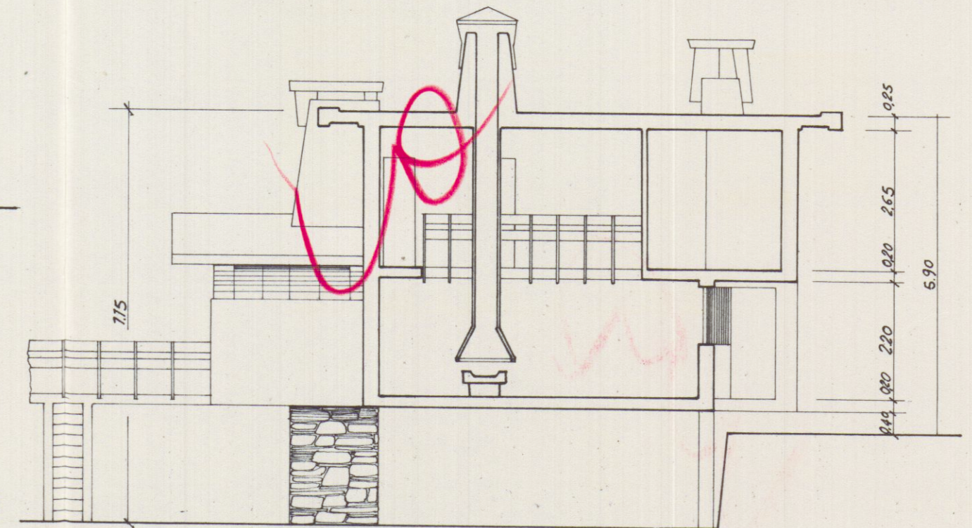
SEZIONE A-B — RAPP. 1:100
