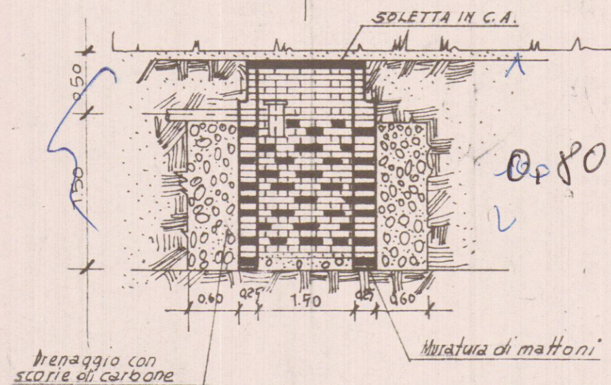
SEZIONE A-B
