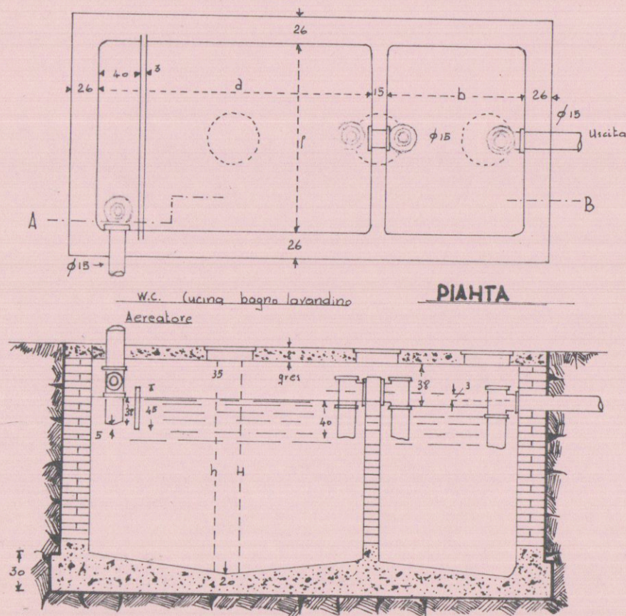
SEZIONE A-B
