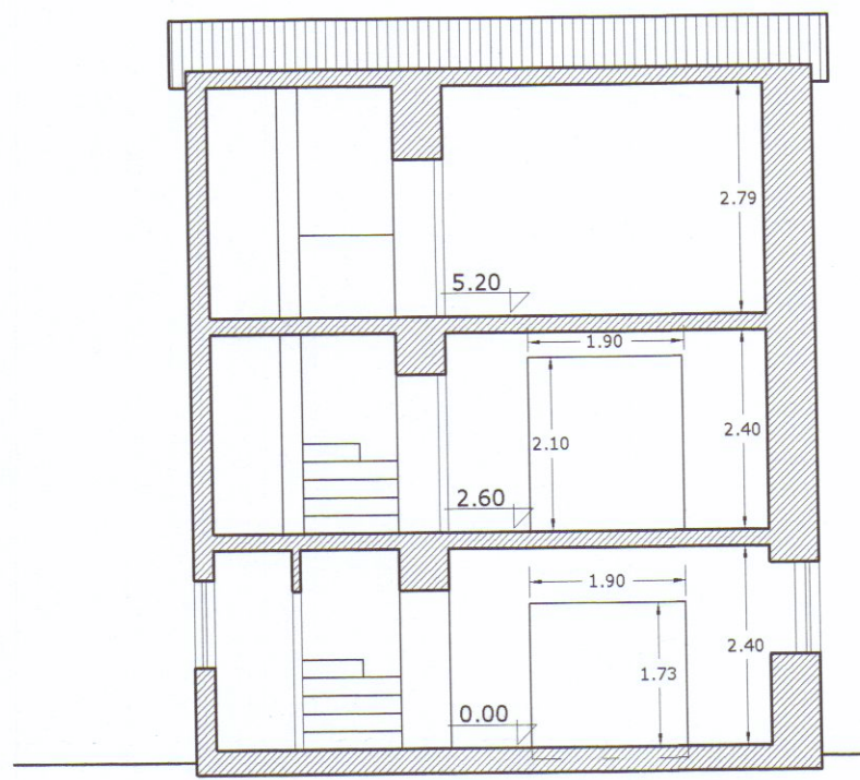
Sezione B-B'
