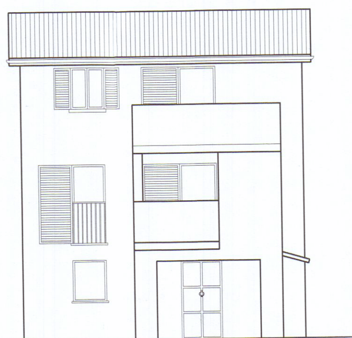
Prospetto est
