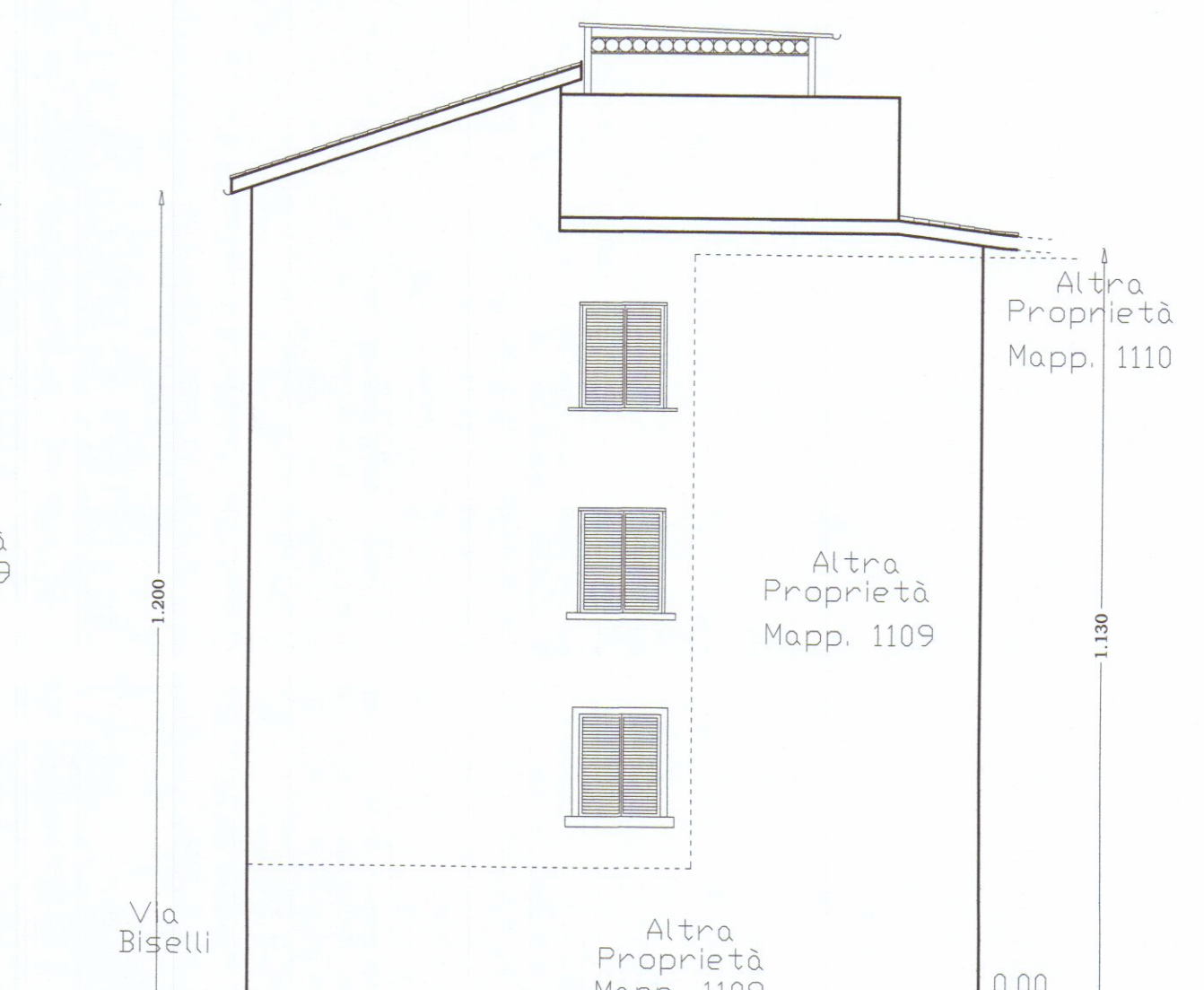
PROSPETTO SUD - EST
