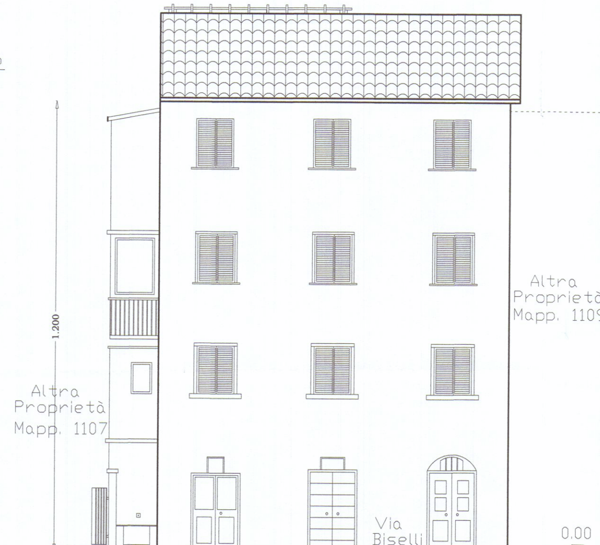
PROSPETTO SUD - OVEST
