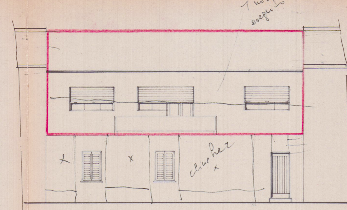
PROSPETTO Via Marco Polo
