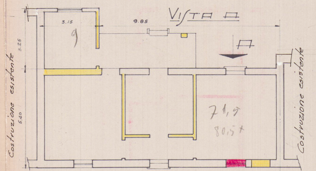
PROGETTO ESISTENTE - Pianta -
