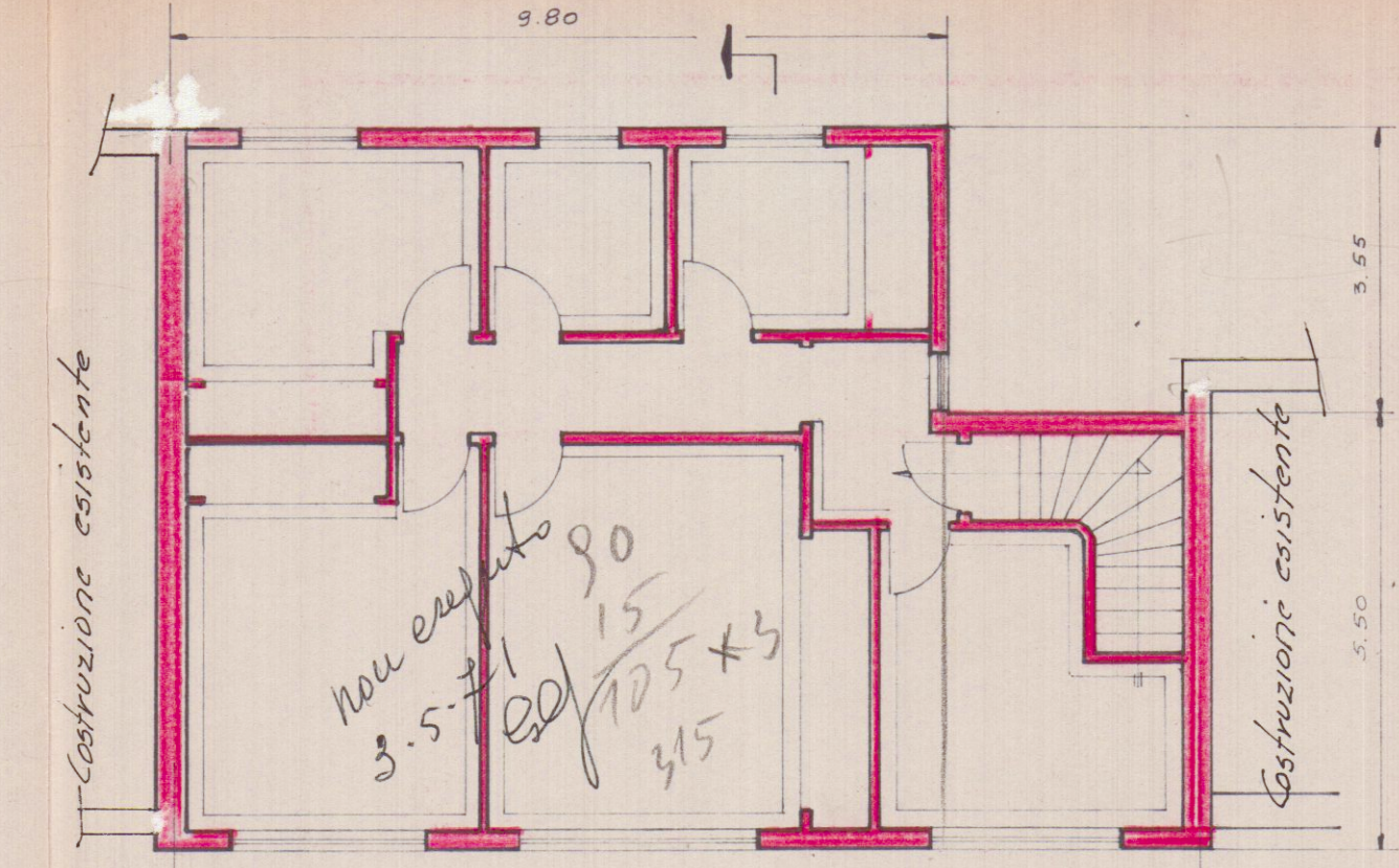
PRIMO PIANO
