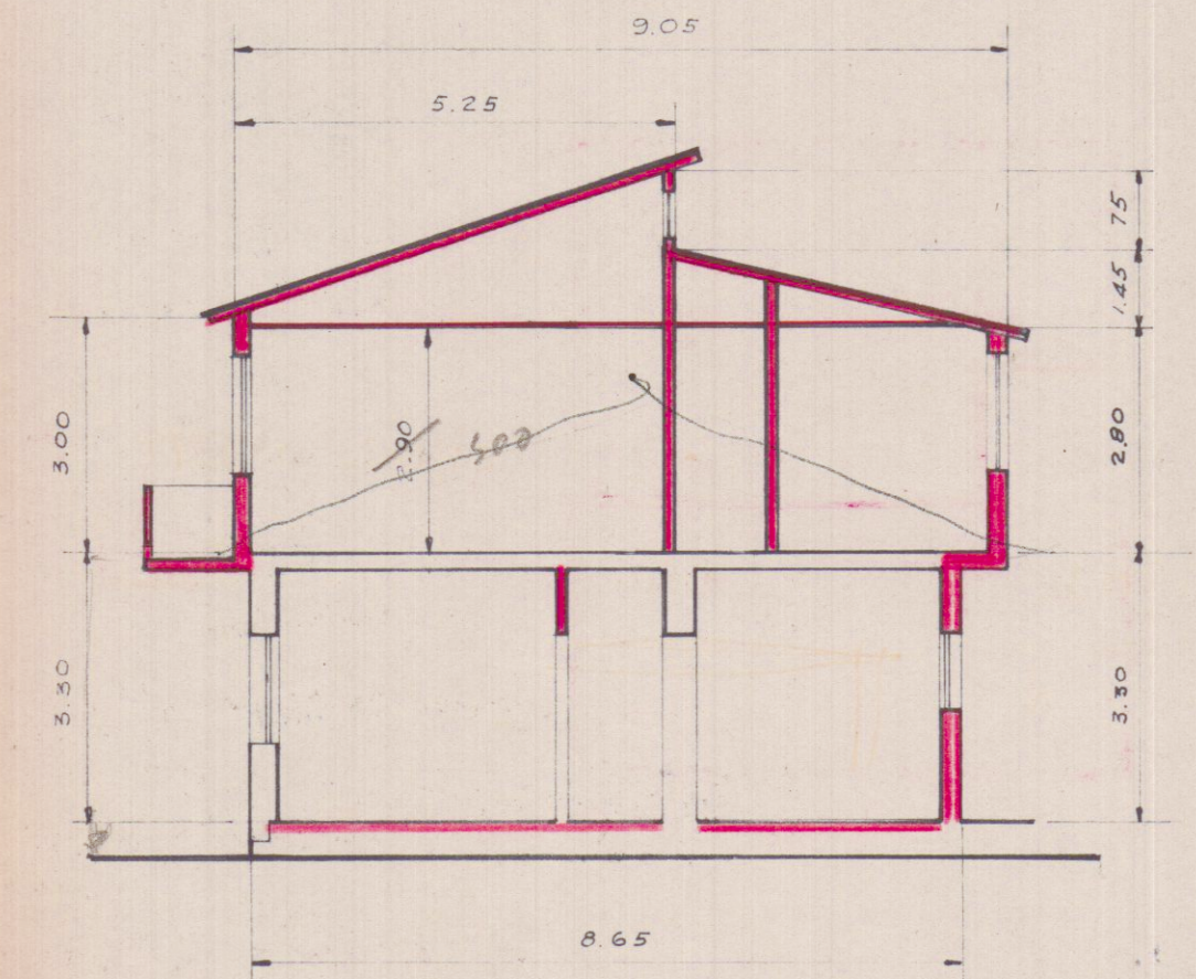
SEZIONE
