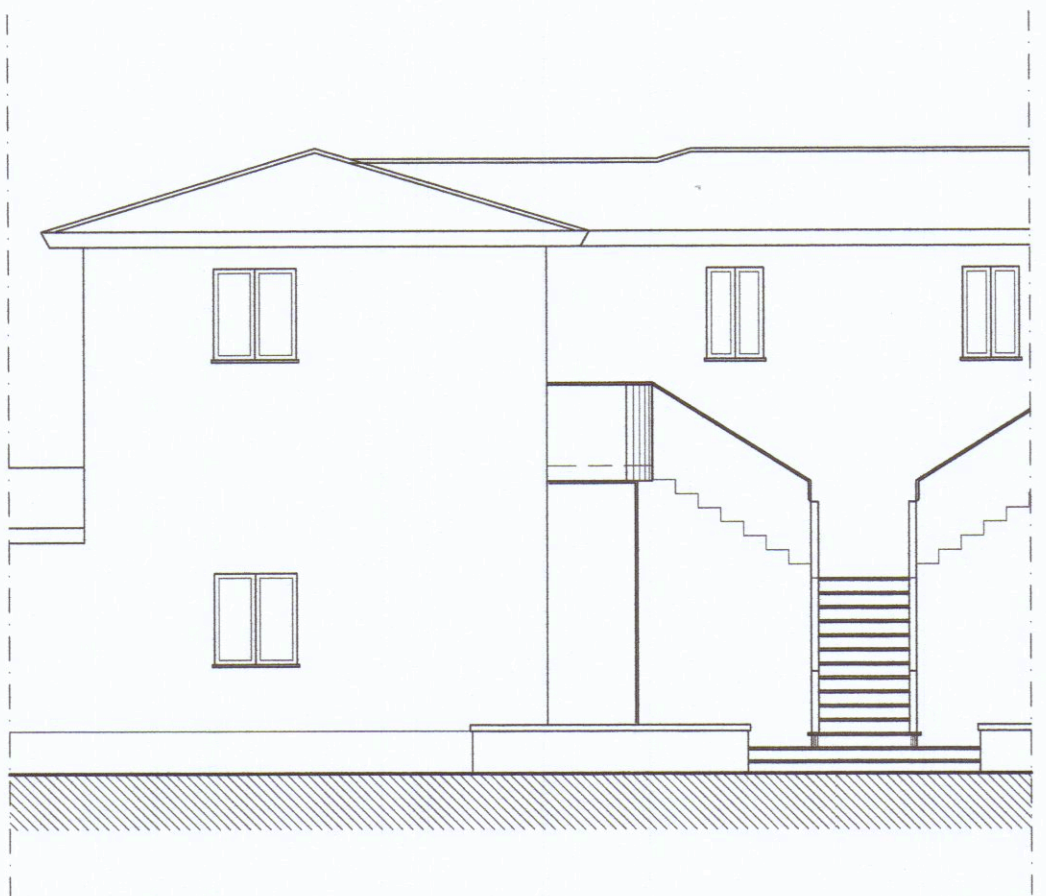
Prospetto SUD
