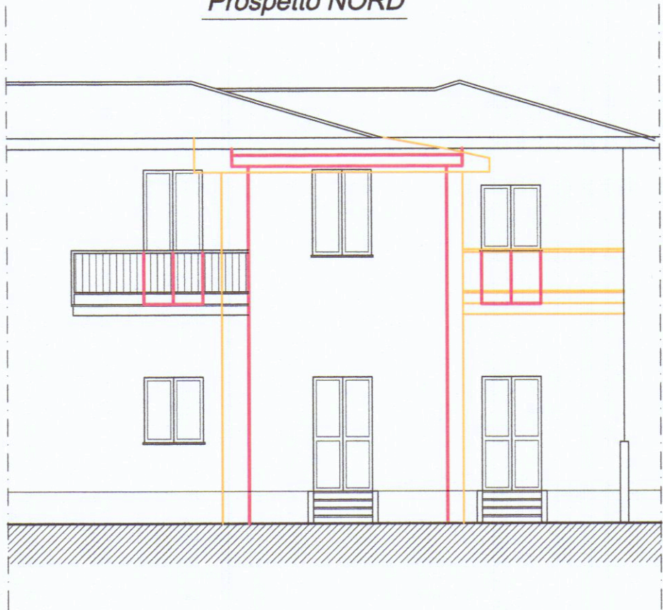
Prospetto NORD
