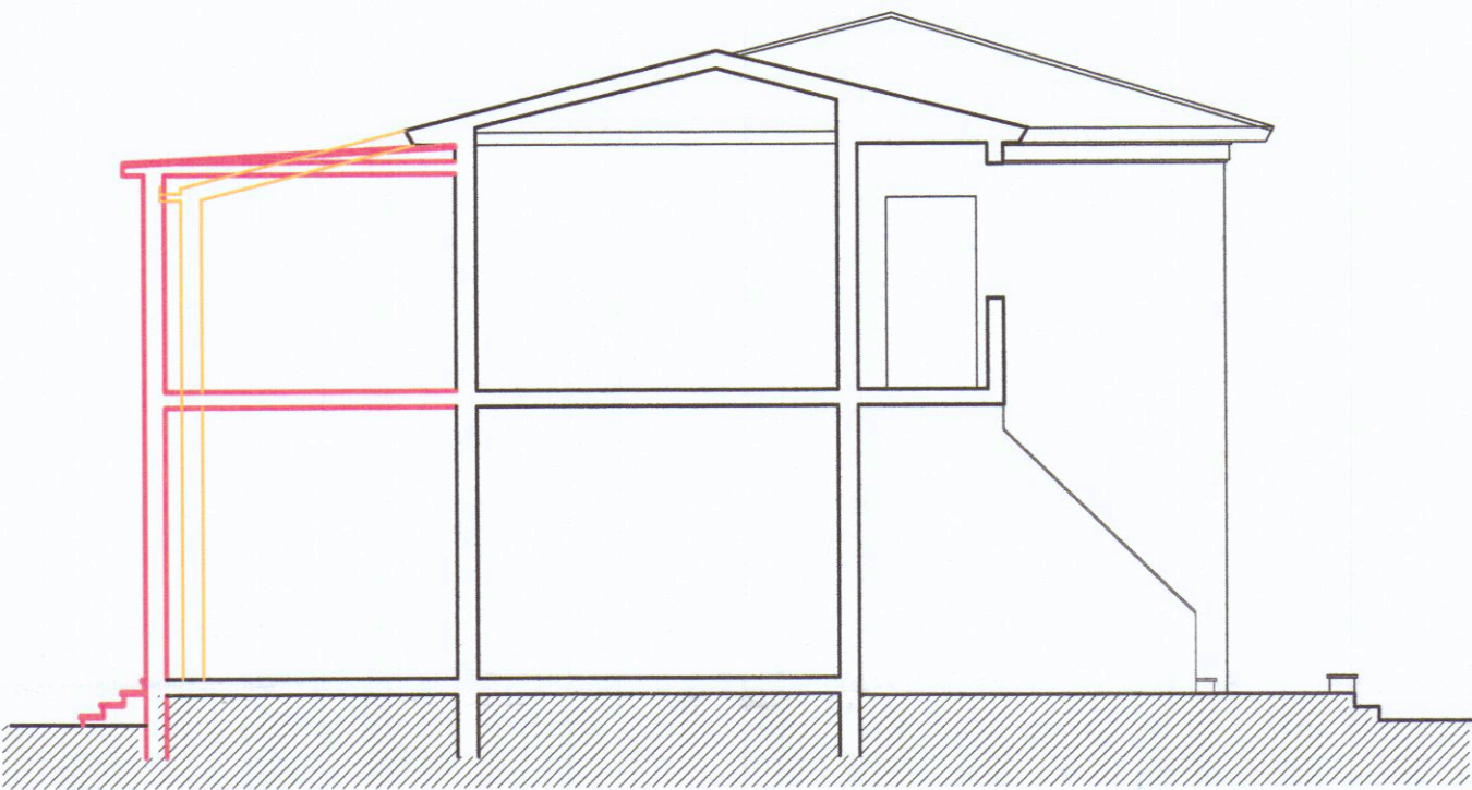
Sezione A-A
