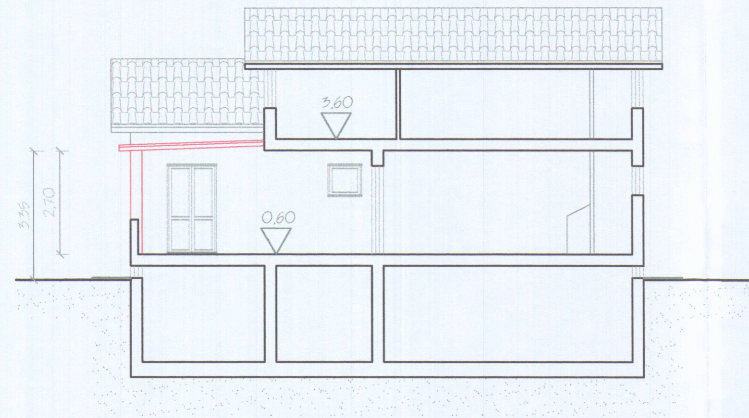
Sezione A-A'
