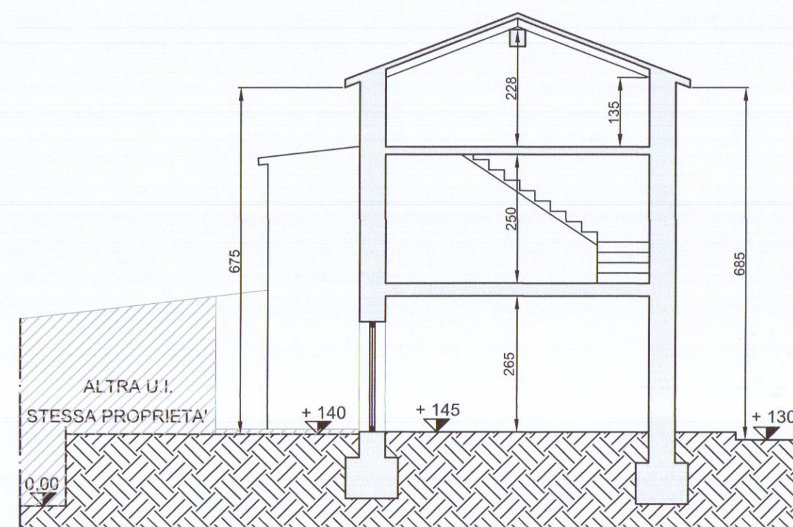
SEZIONE B-B
