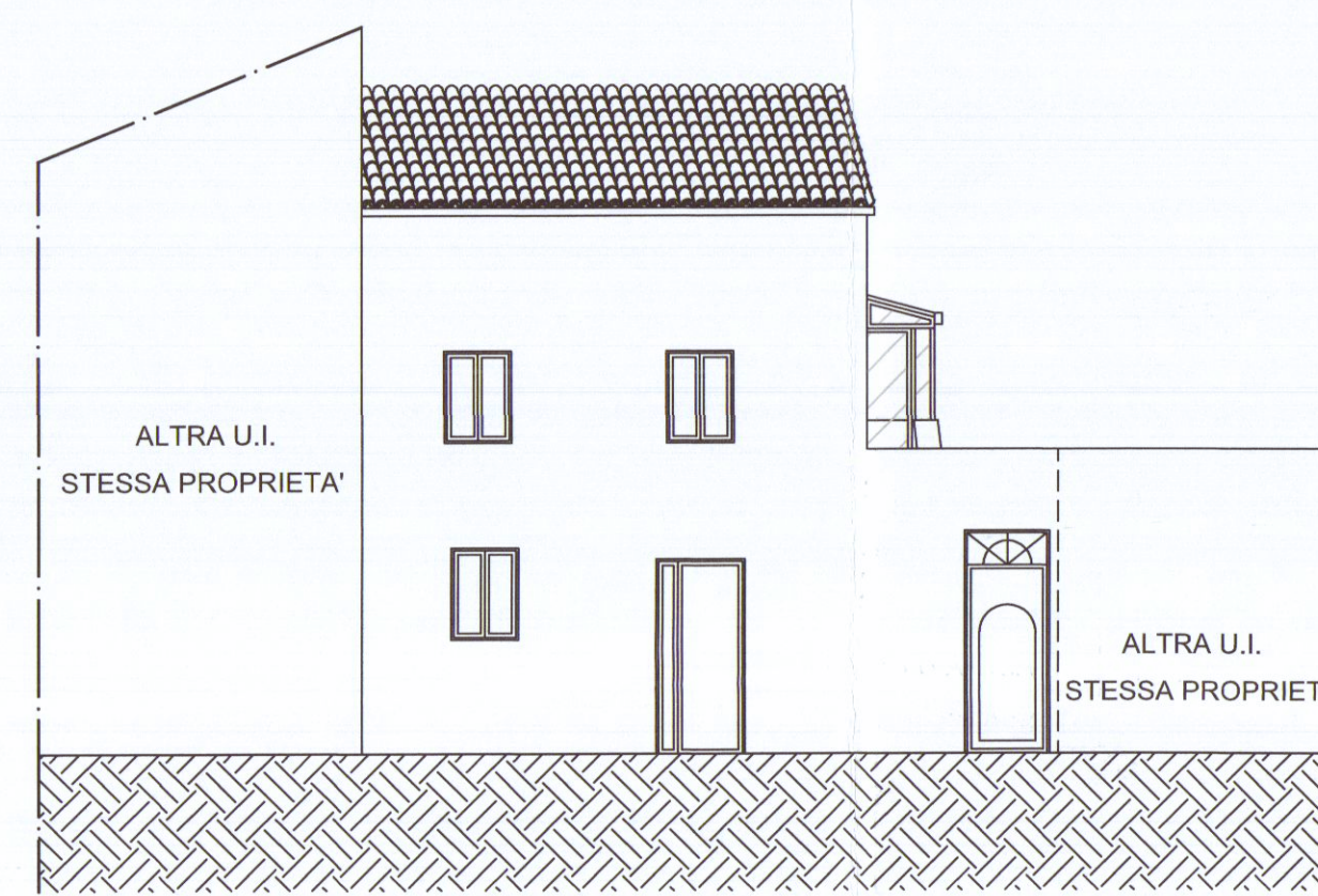
PROSPETTO NORD EST
