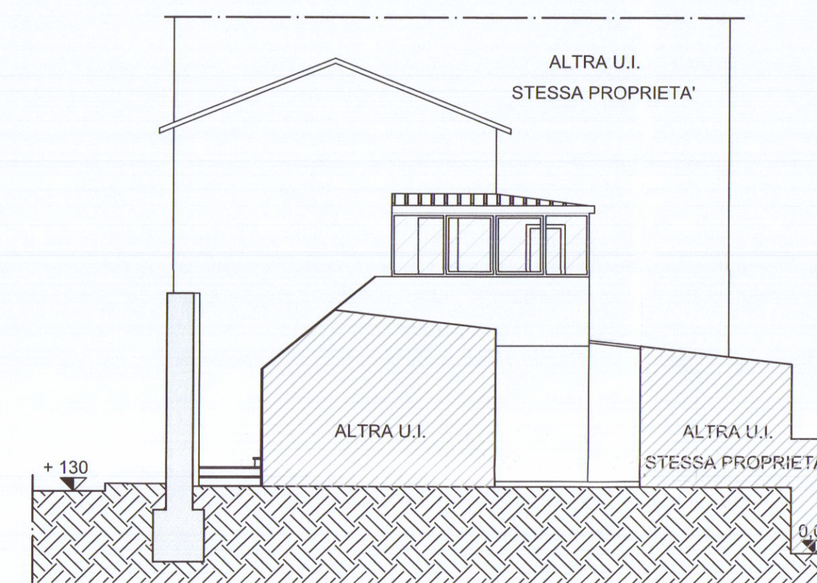
PROSPETTO OVEST
