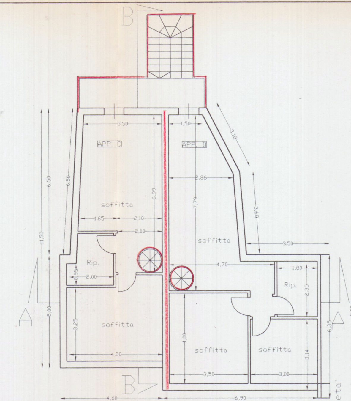
PIANO SOTTOTETTO
