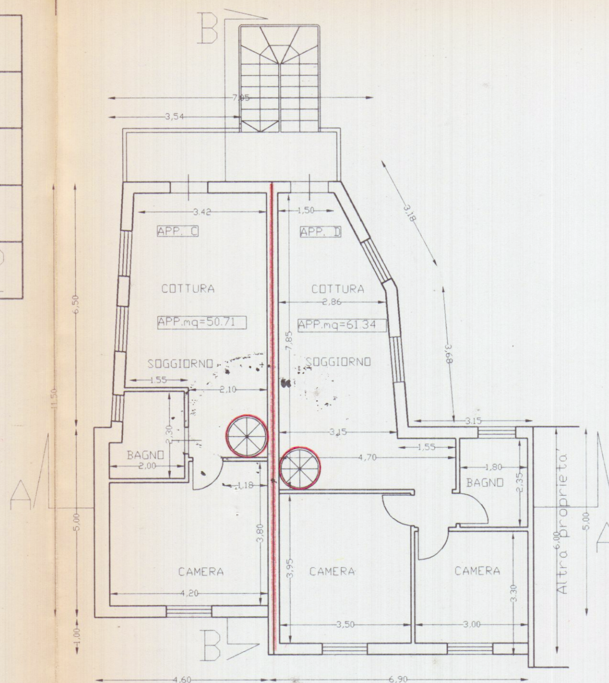
PIANO PRIMO
