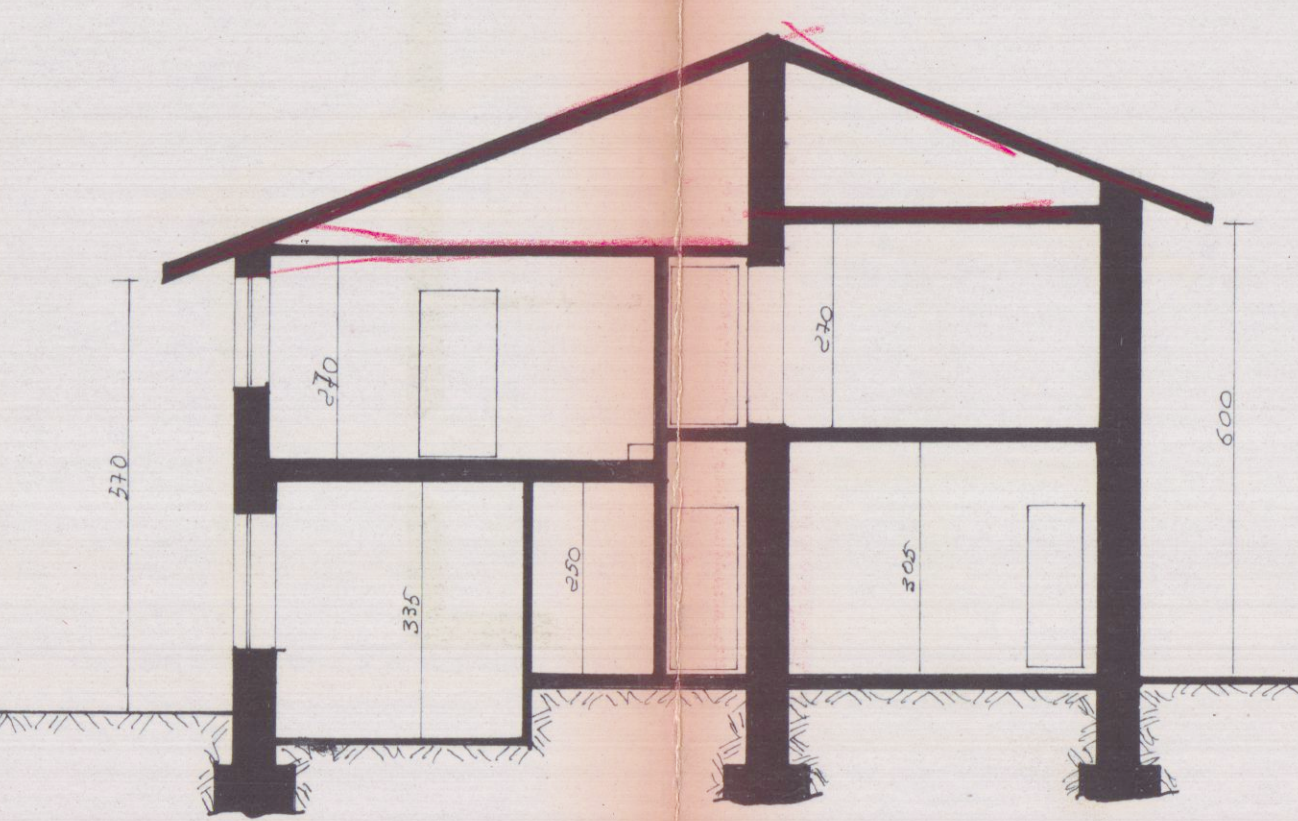
SEZIONE A-A
