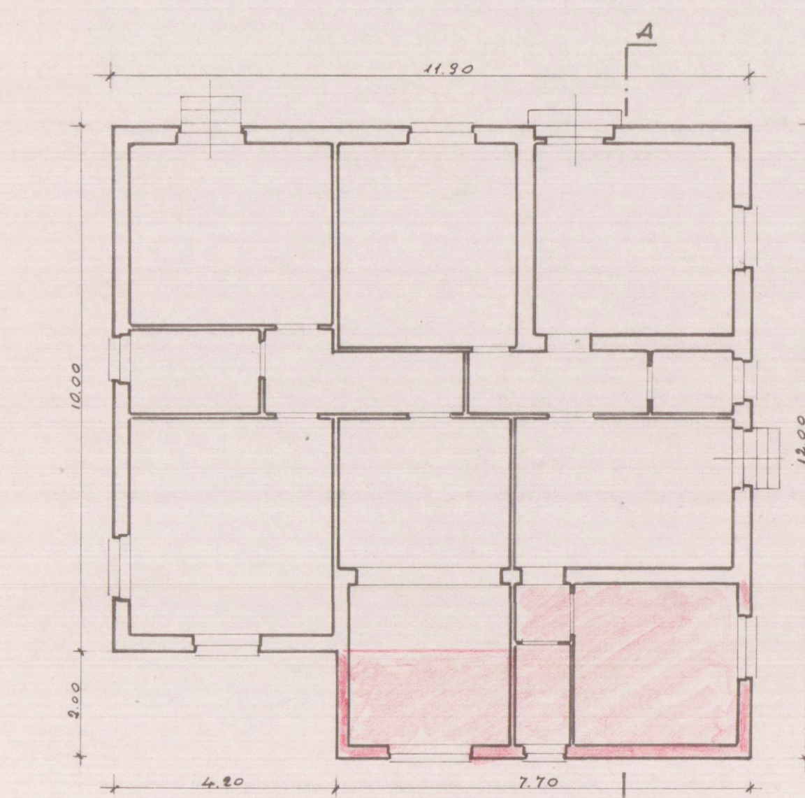
PIANTA
