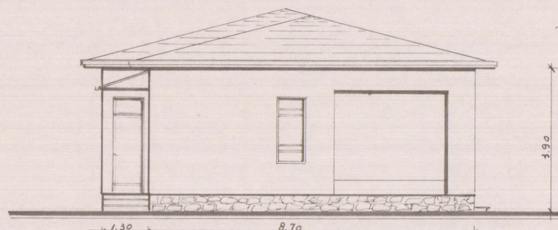
PROSPETTO LEVANTE
