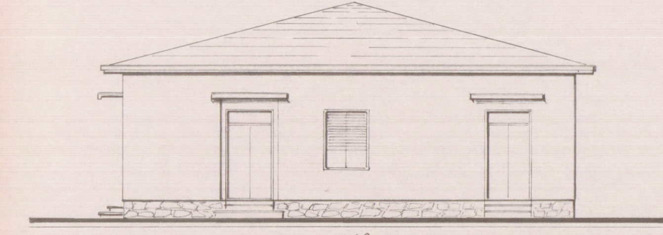
PROSPETTO STRADA
