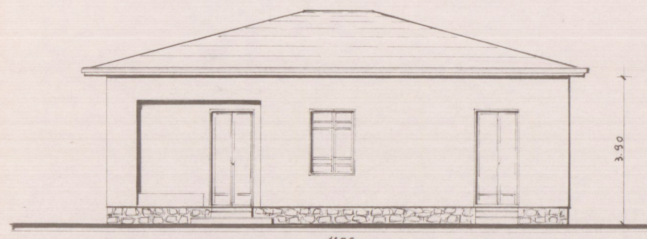
PROSPETTO STRADA
