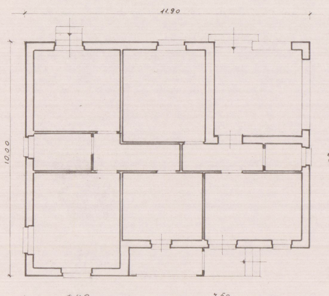
PIANTA
