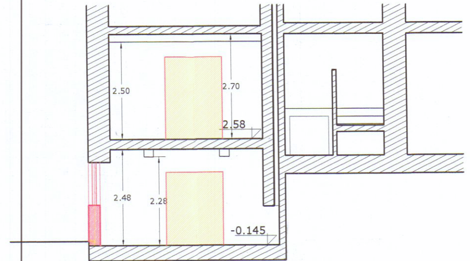
Sezione A-A'
