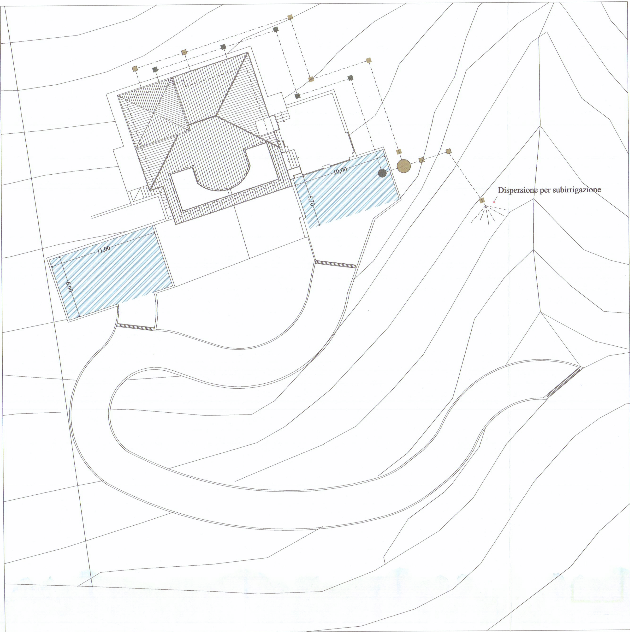
SISTEMAZIONE ESTERNA DI PROGETTO - zone a parcheggio scala 1/200
