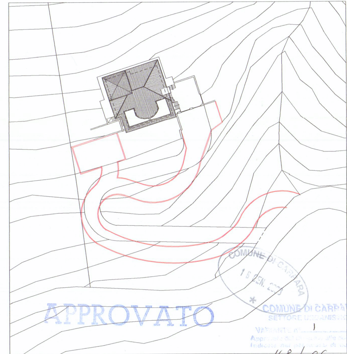
SISTEMAZIONE ESTERNA DI RAFFRONTO scala 1/500
