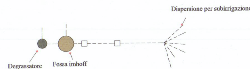
SISTEMAZIONE ESTERNA DI PROGETTO scala 1/500
