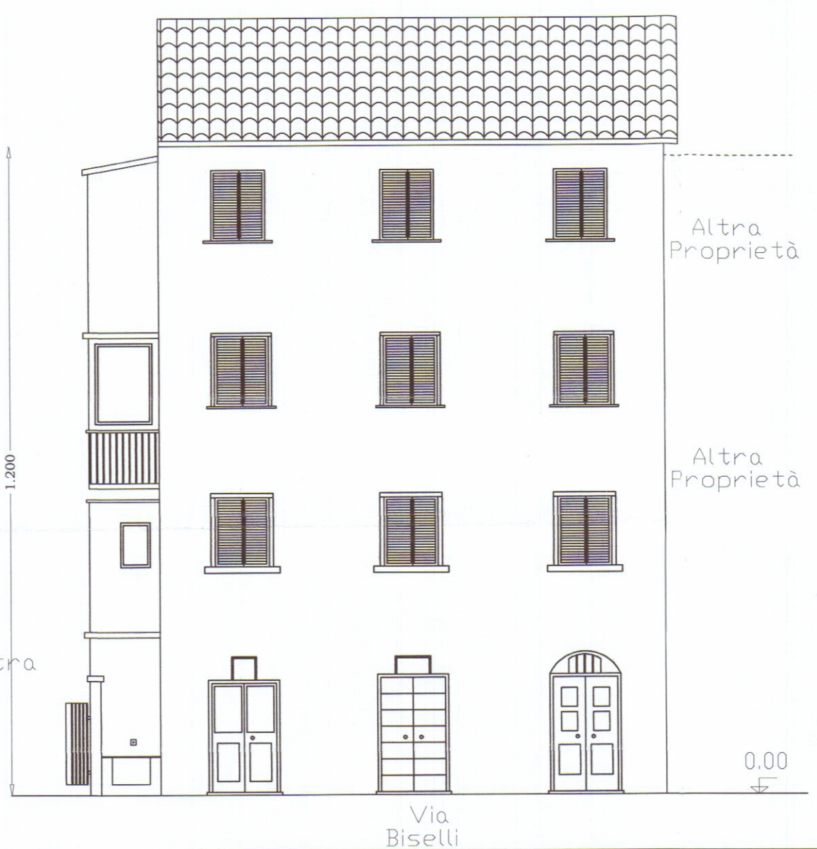
PROSPETTO SUD - OVEST
