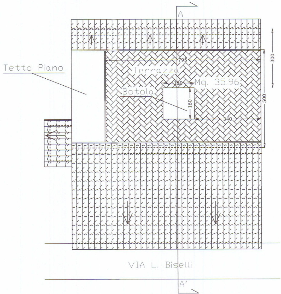
Pianta Copertura
