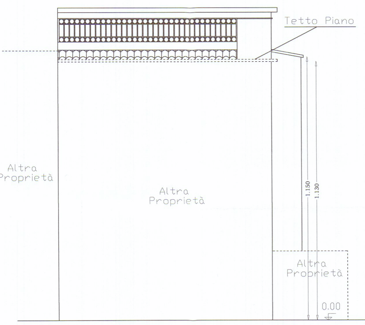
PROSPETTO NORD - EST
