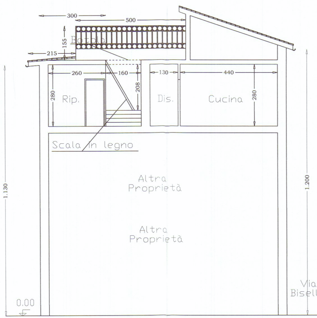
Sezione A-A'
