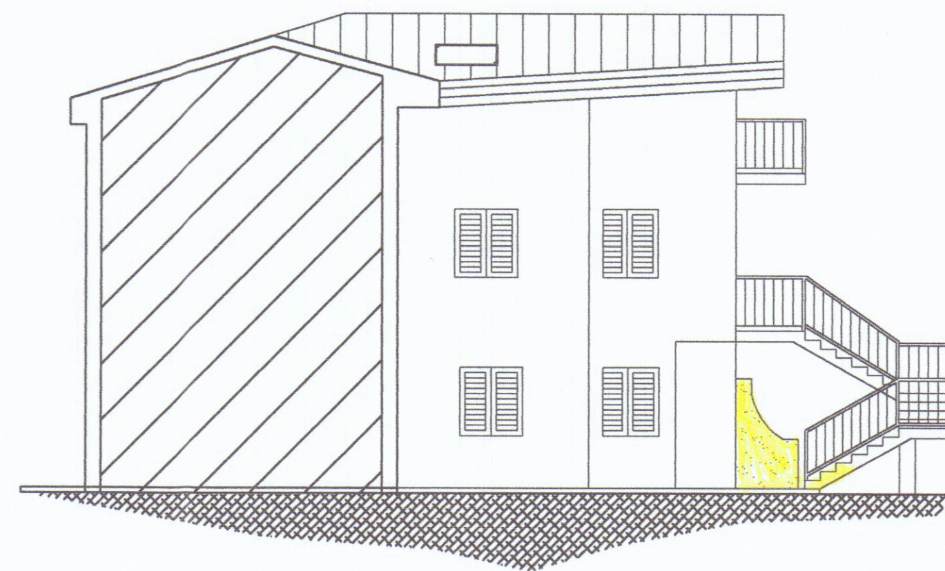
PROSPETTO OVEST
