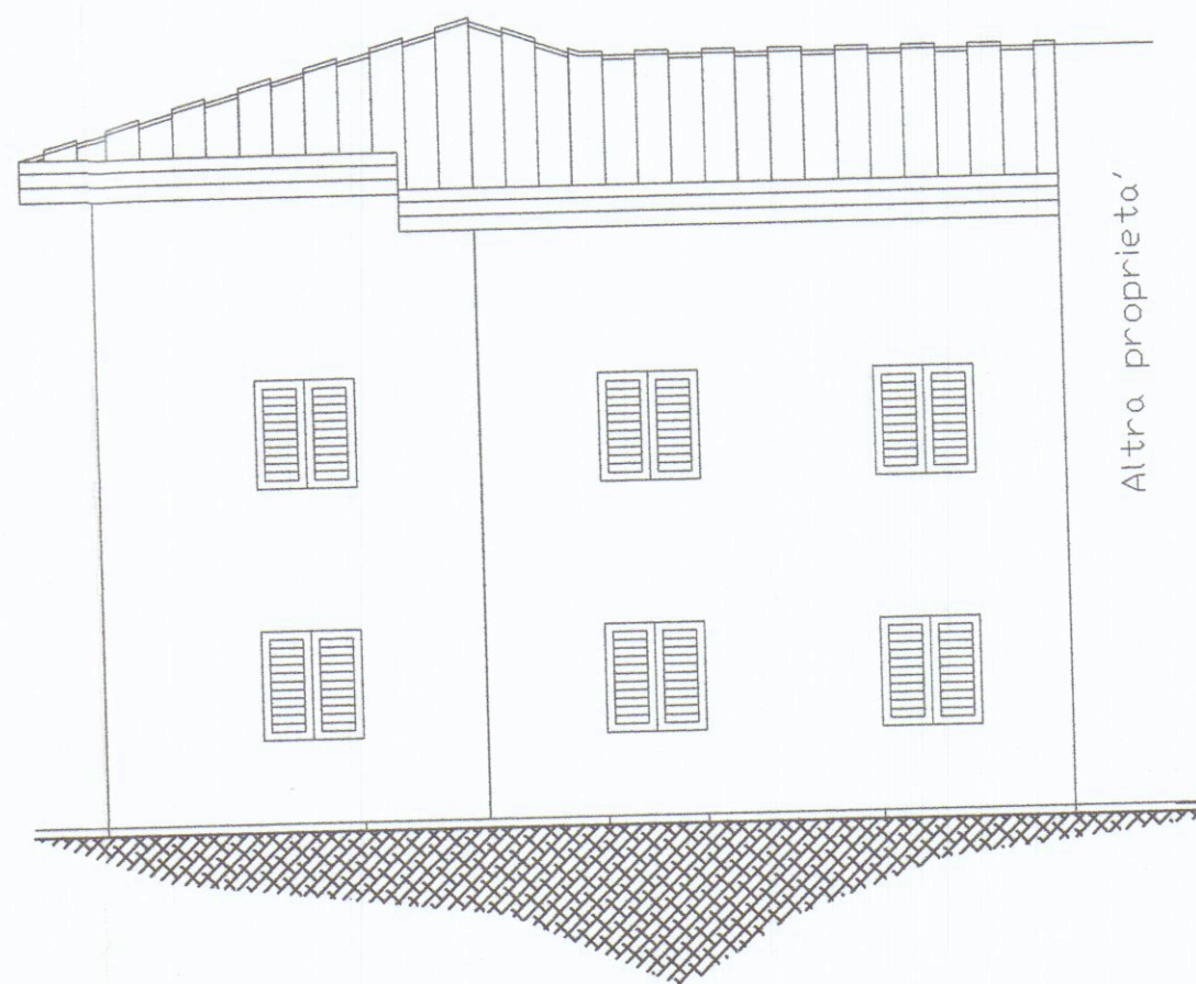
PROSPETTO NORD
