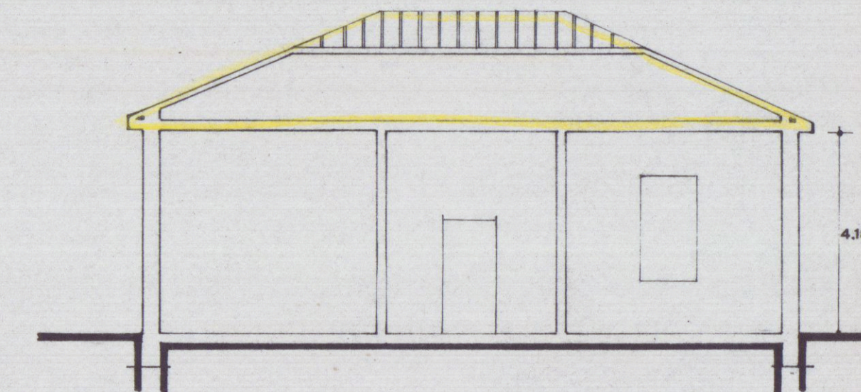
SEZIONE A-A
