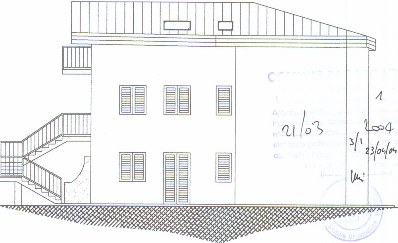
PROSPETTO EST
