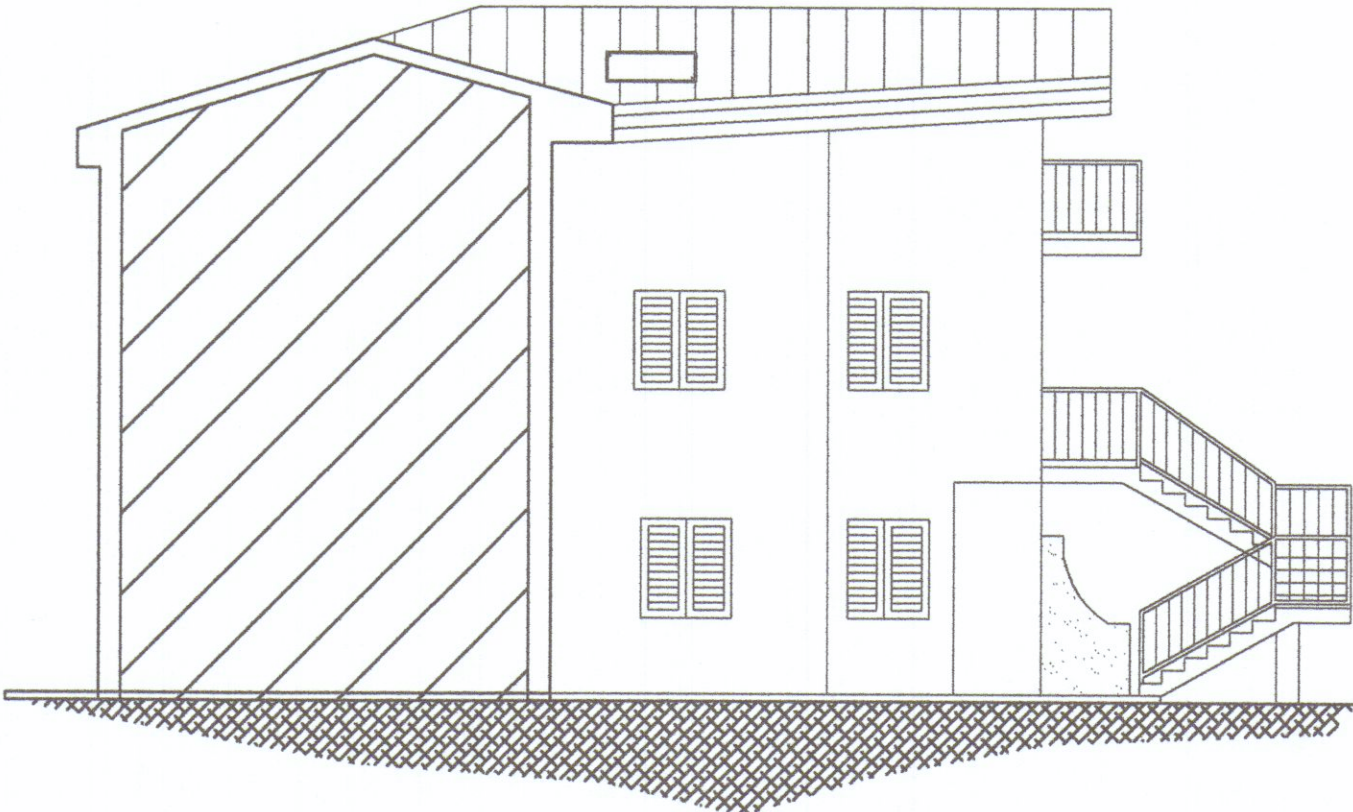
PROSPETTO OVEST
