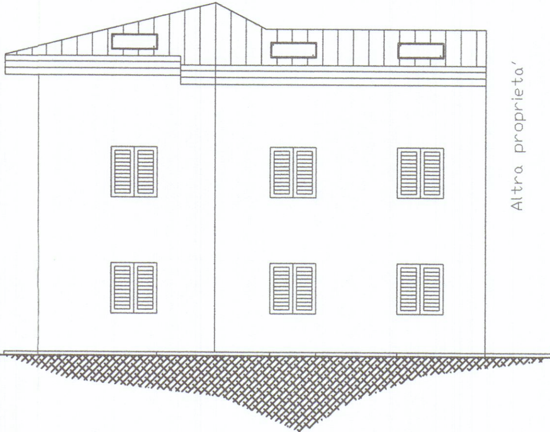
PROSPETTO NORD
