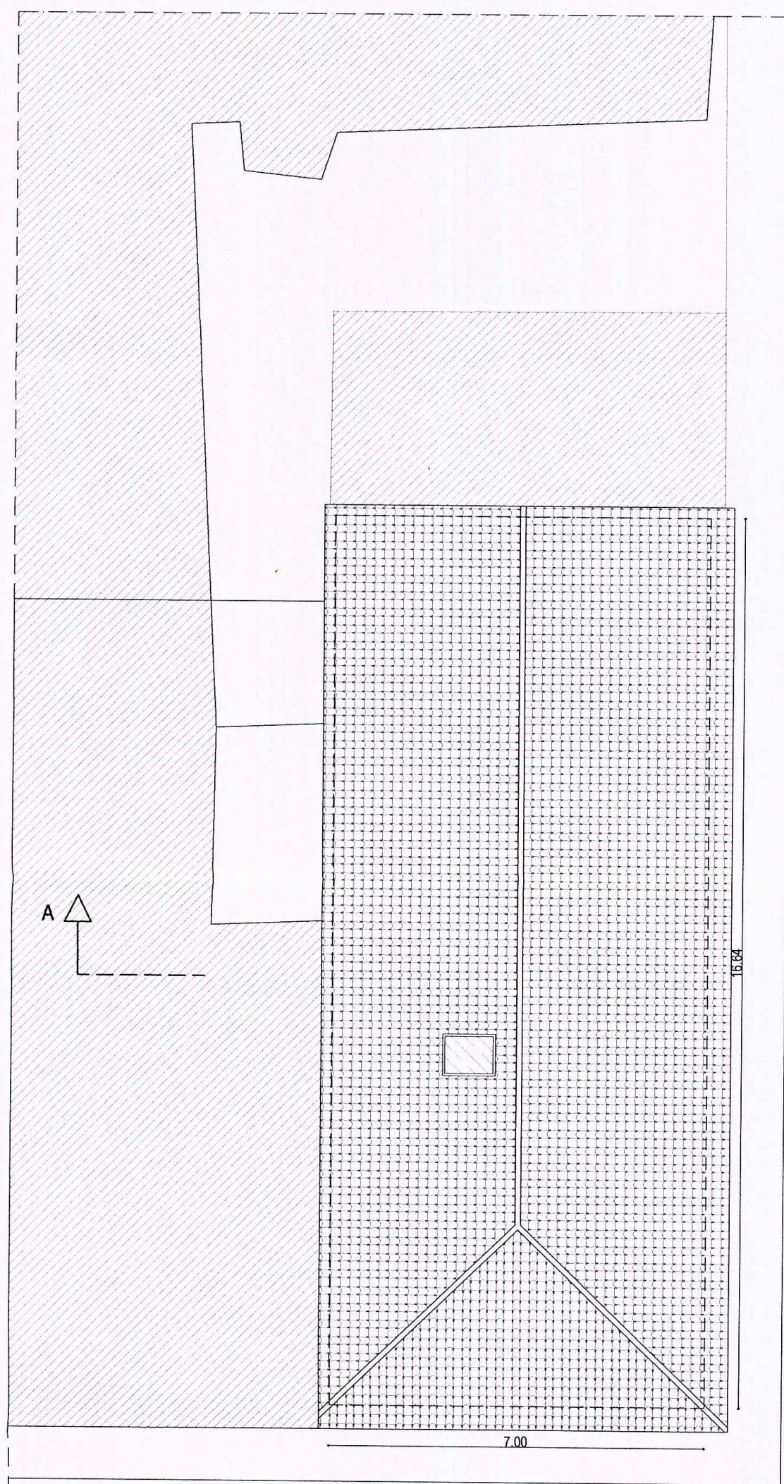
PIANTA DELLA COPERTURA
