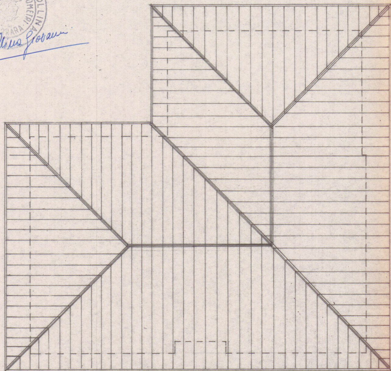
PIANTA TETTO
