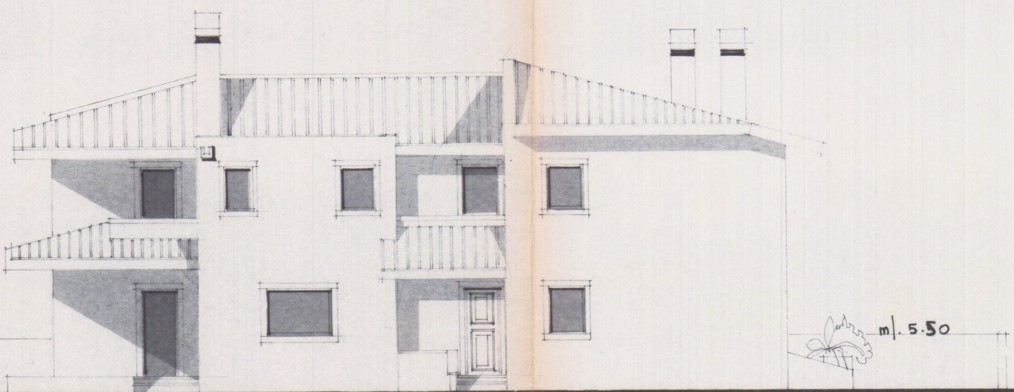
PROSPETTO OVEST
