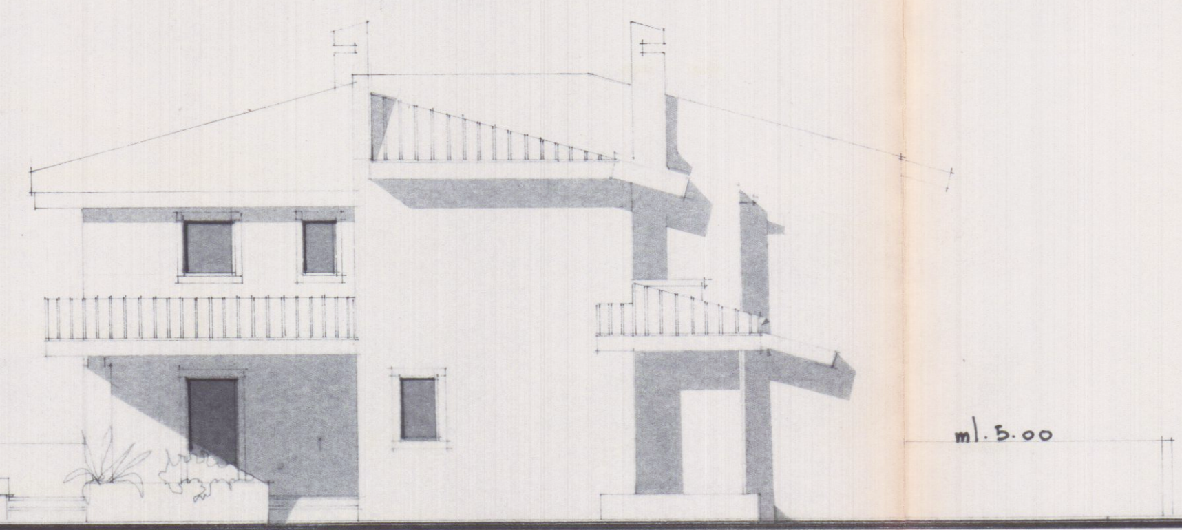
PROSPETTO NORD
