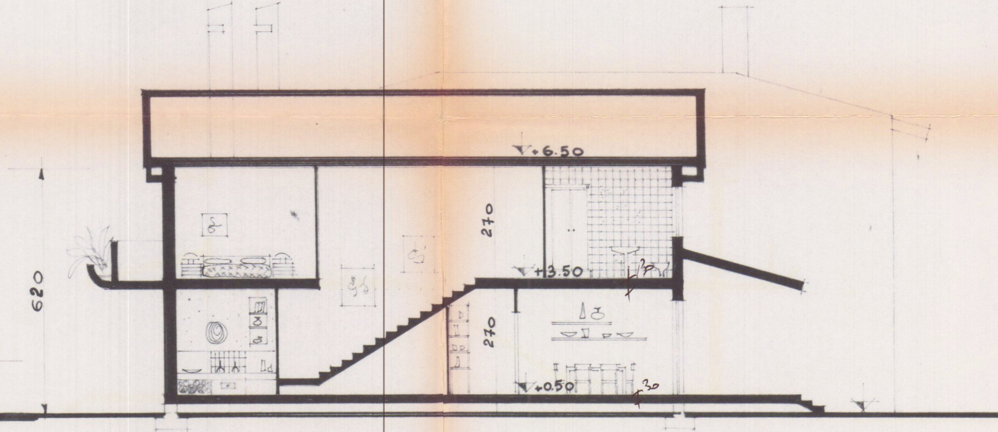
SEZIONE LONG.
