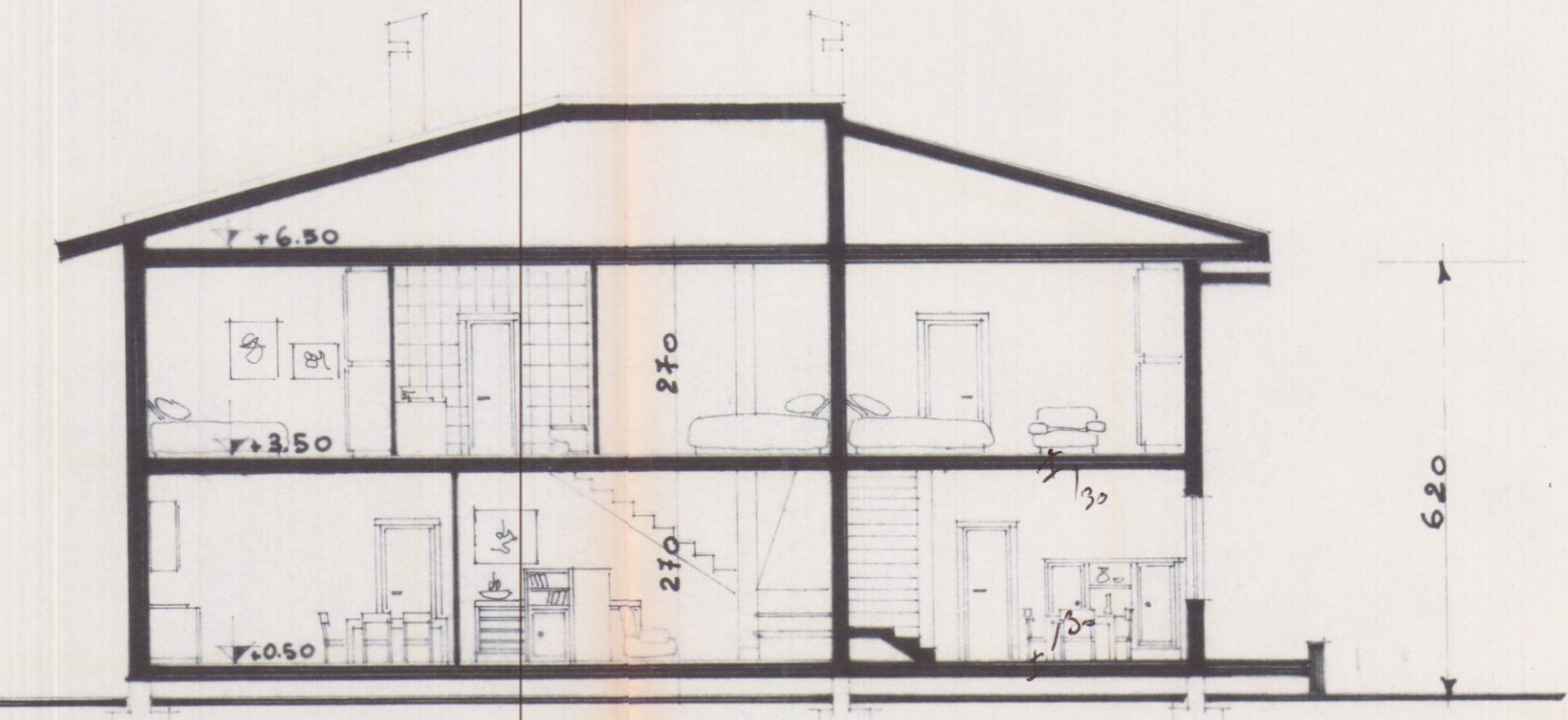
SEZIONE TRASV.
