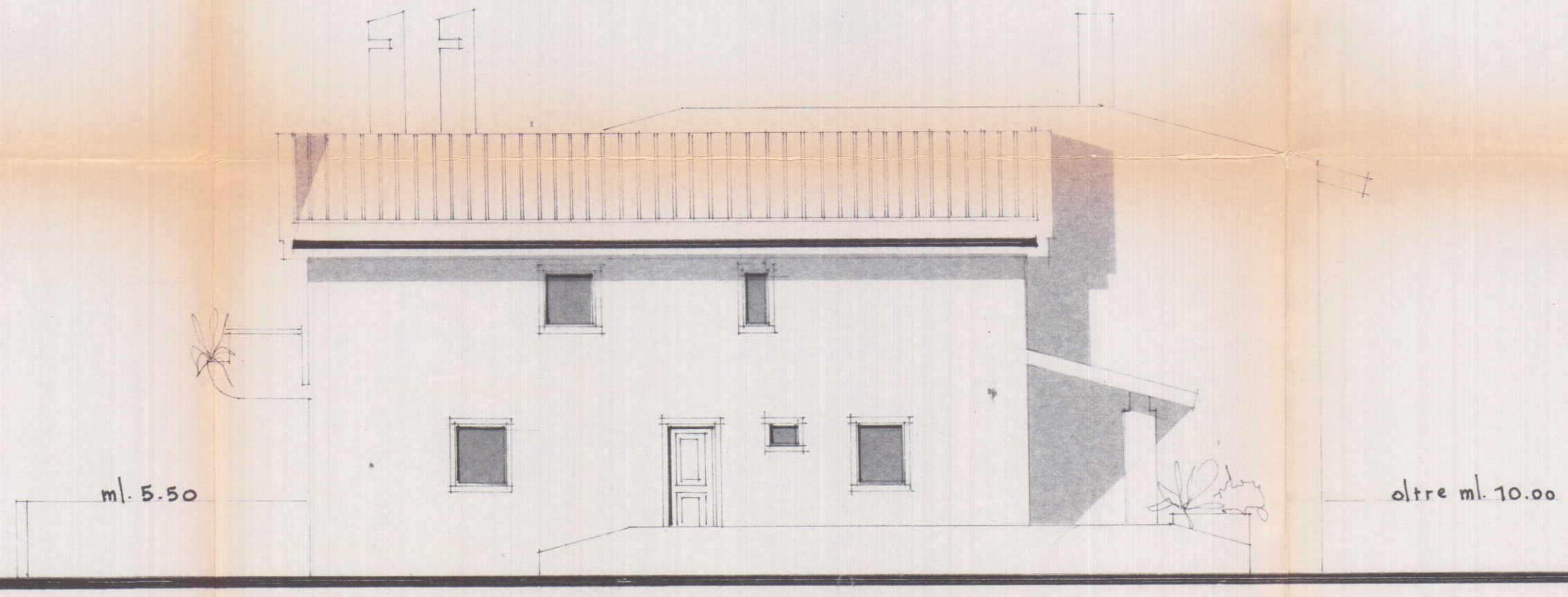
PROSPETTO EST
