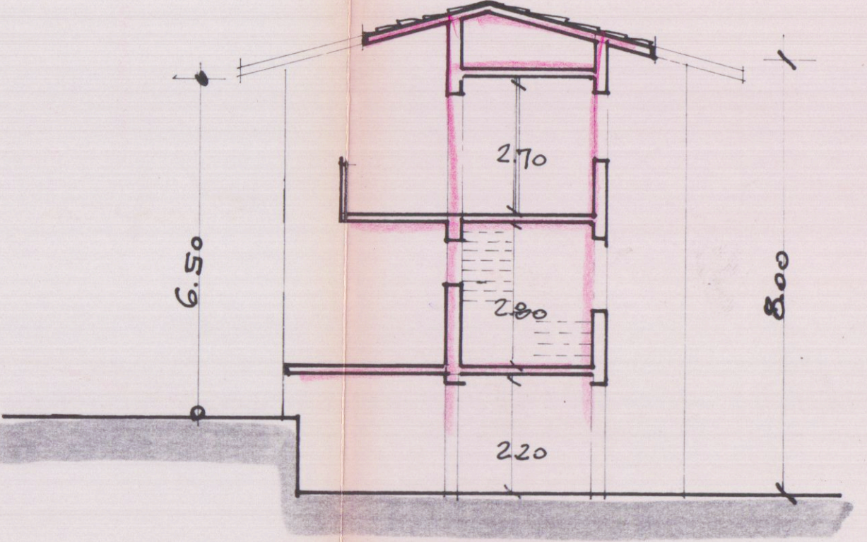
SEZIONE
