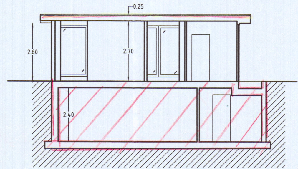
Sezione ZZ''
