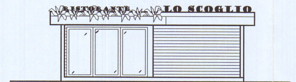
Prospetto Sud-Ovest
