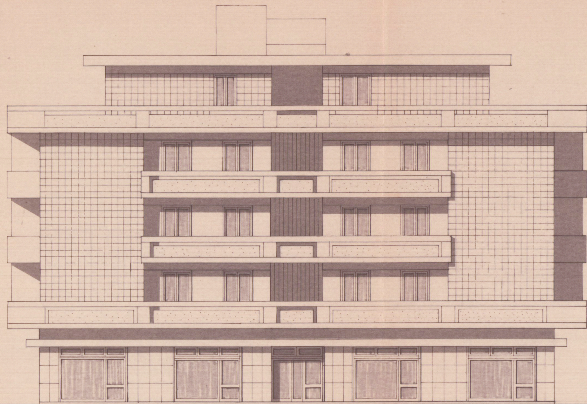
PROSPETTO NORD
