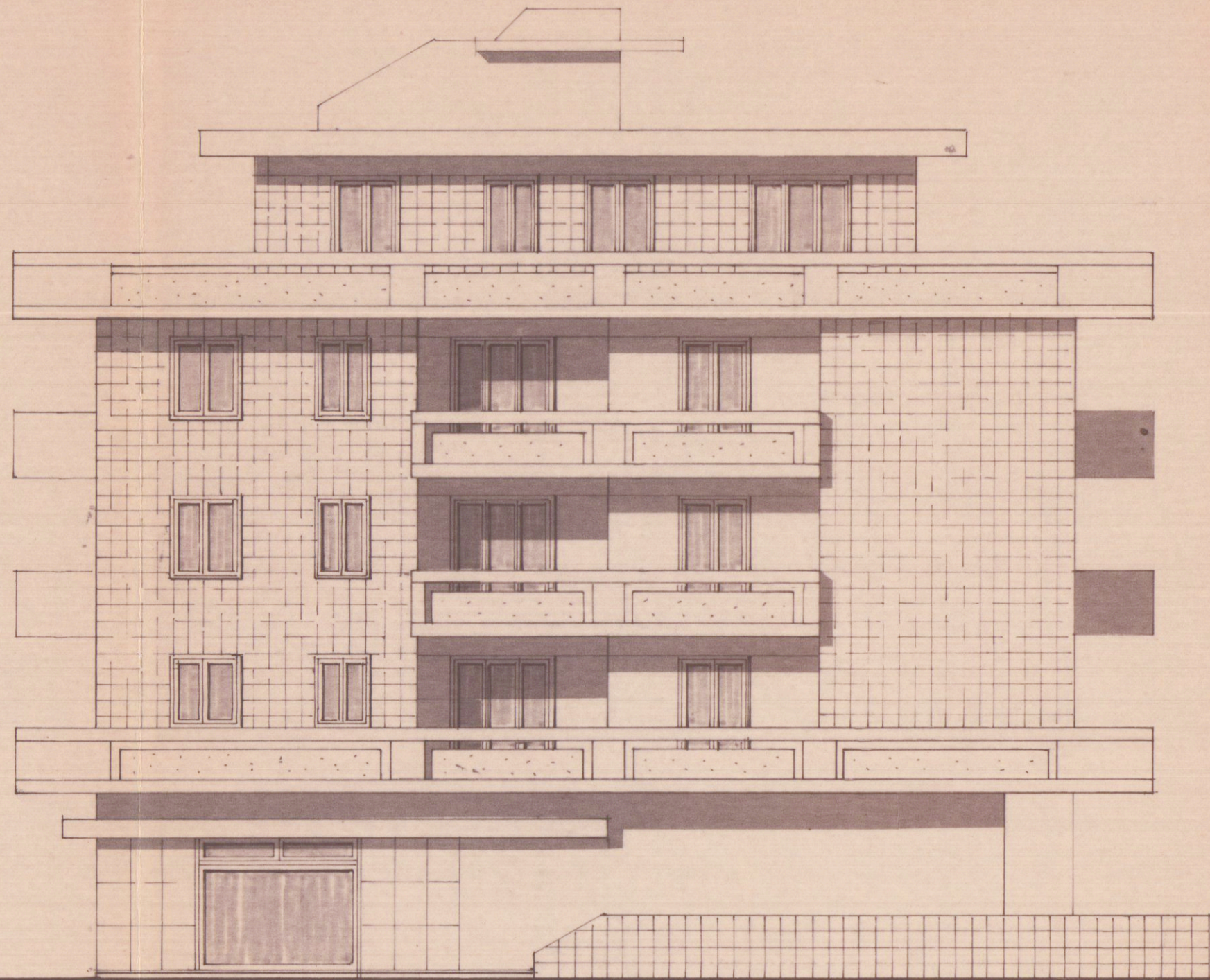
PROSPETTO OVEST
