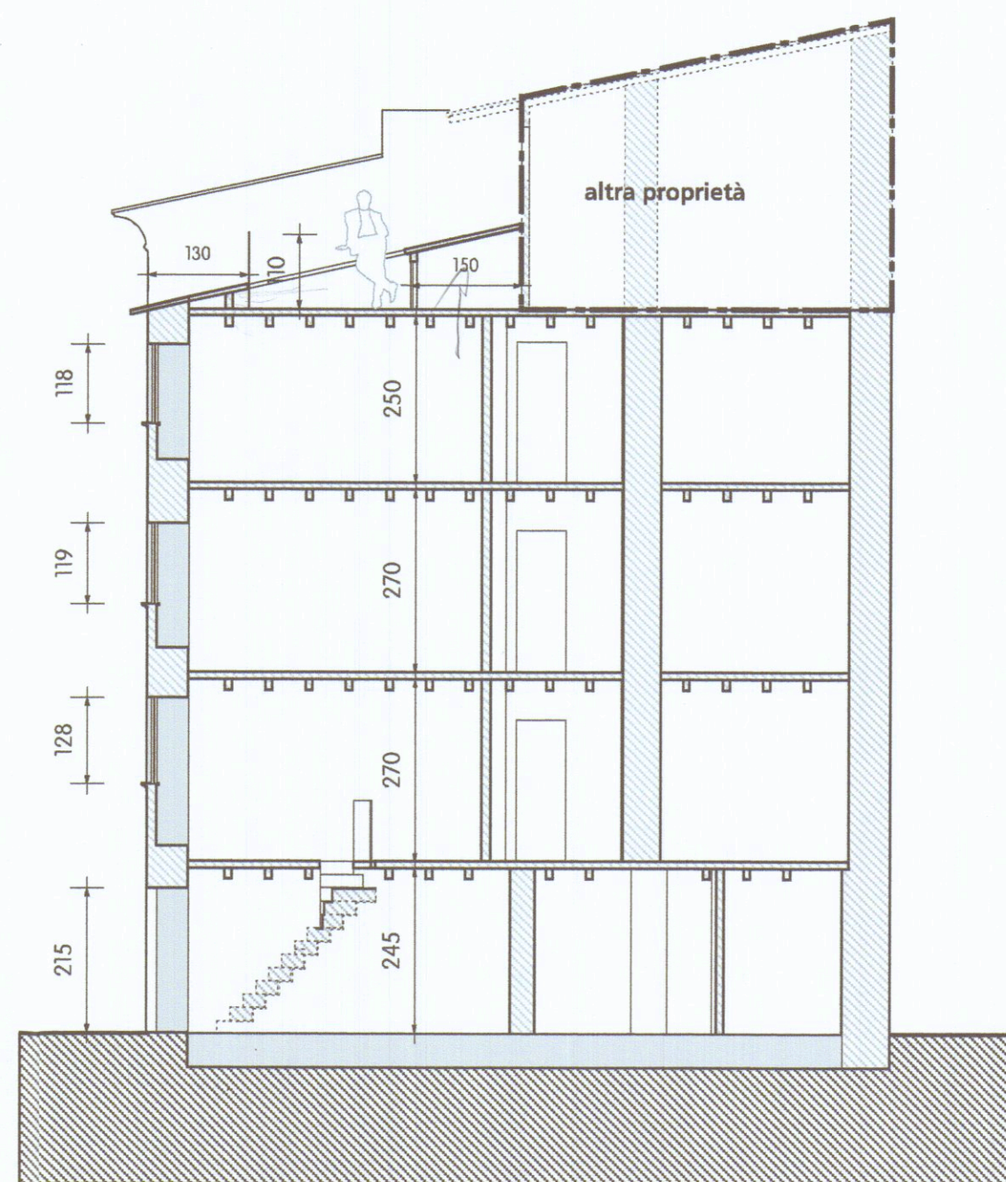
6 sezione scala 1: 100
