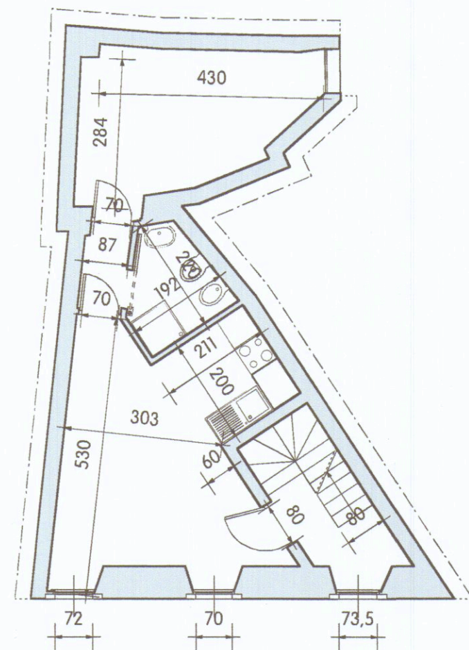
3 piano piano secondo scala 1: 100
