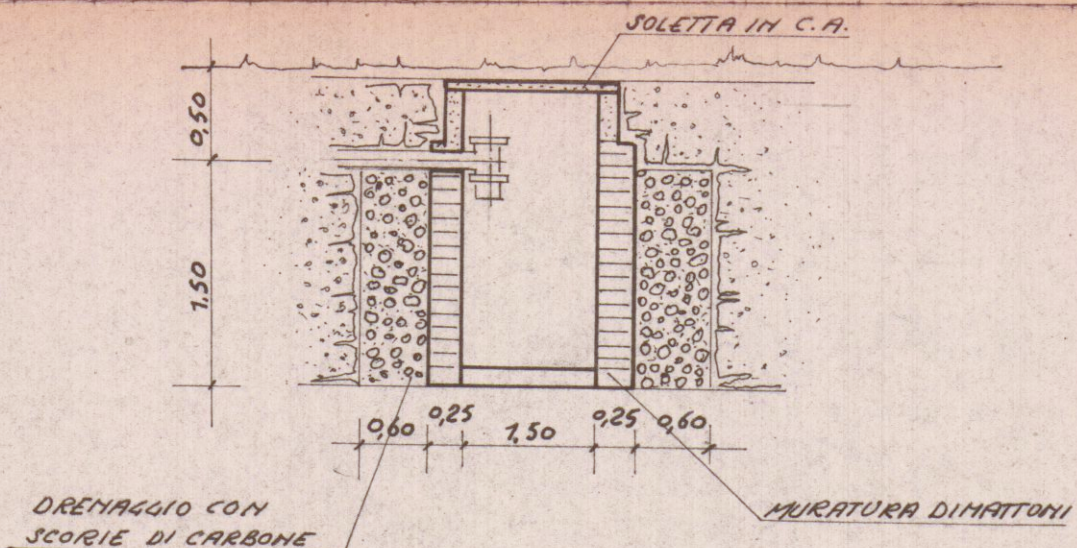
SEZIONE BB
