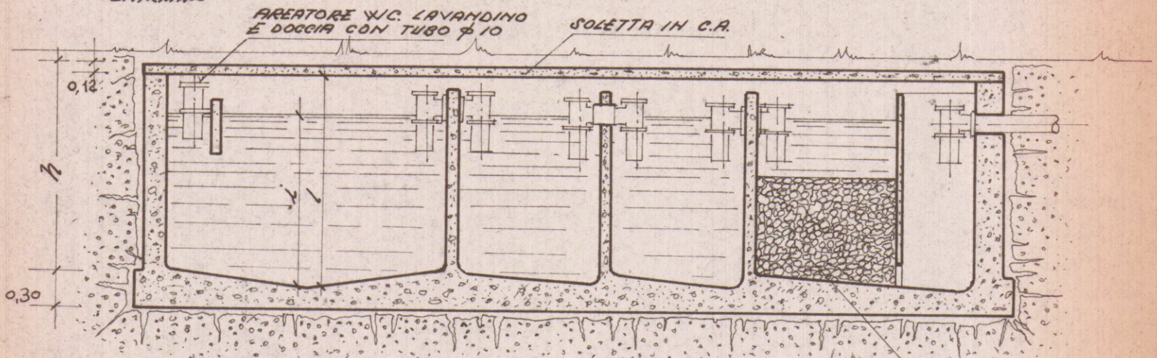
SEZIONE AA
