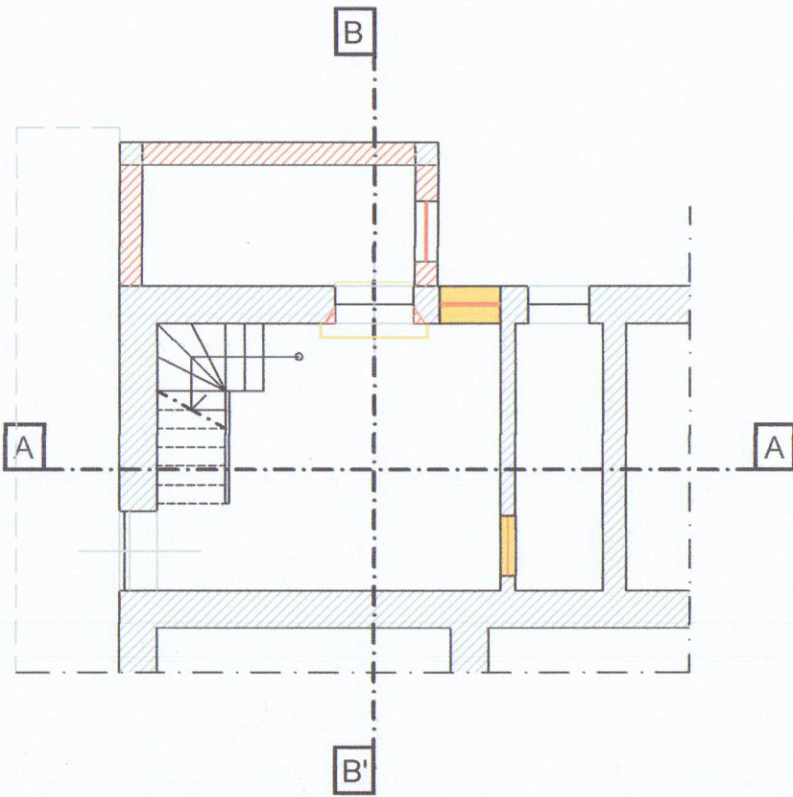
PIANTA PIANO TERRA scala 1.100
