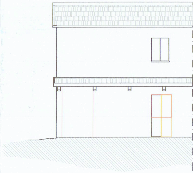
PROSPETTO LATERALE scala 1.100
