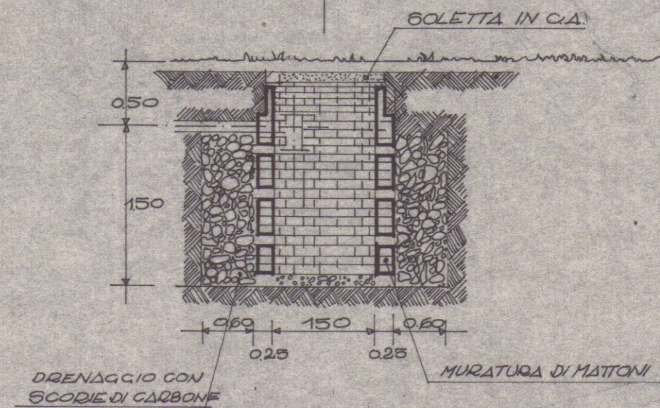
SEZIONE
