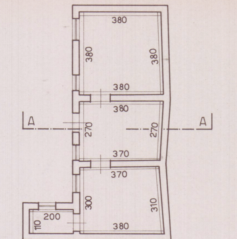
PIANTA LOCALE DI DEPOSITO
