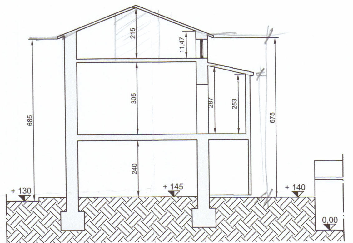
SEZIONE A-A
