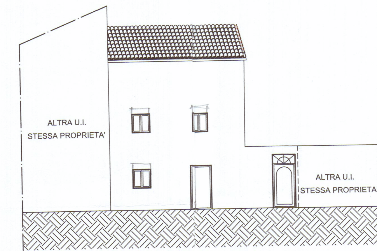
PROSPETTO NORD EST
