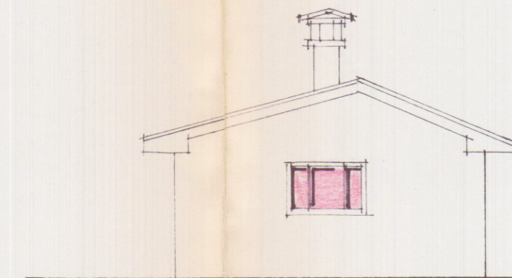
PROSPETTO SUD
