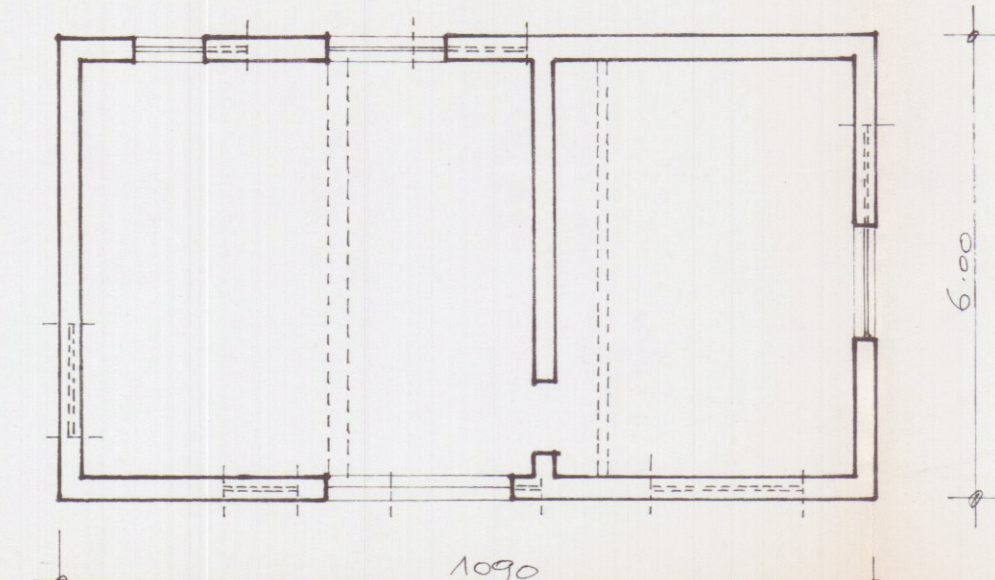
STATO SOVRAPPONTO
