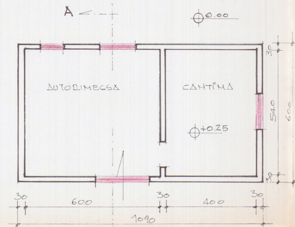
PIANTA MODIFICATA
