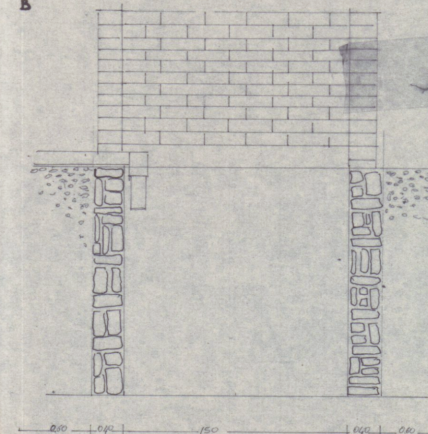
SEZIONE
