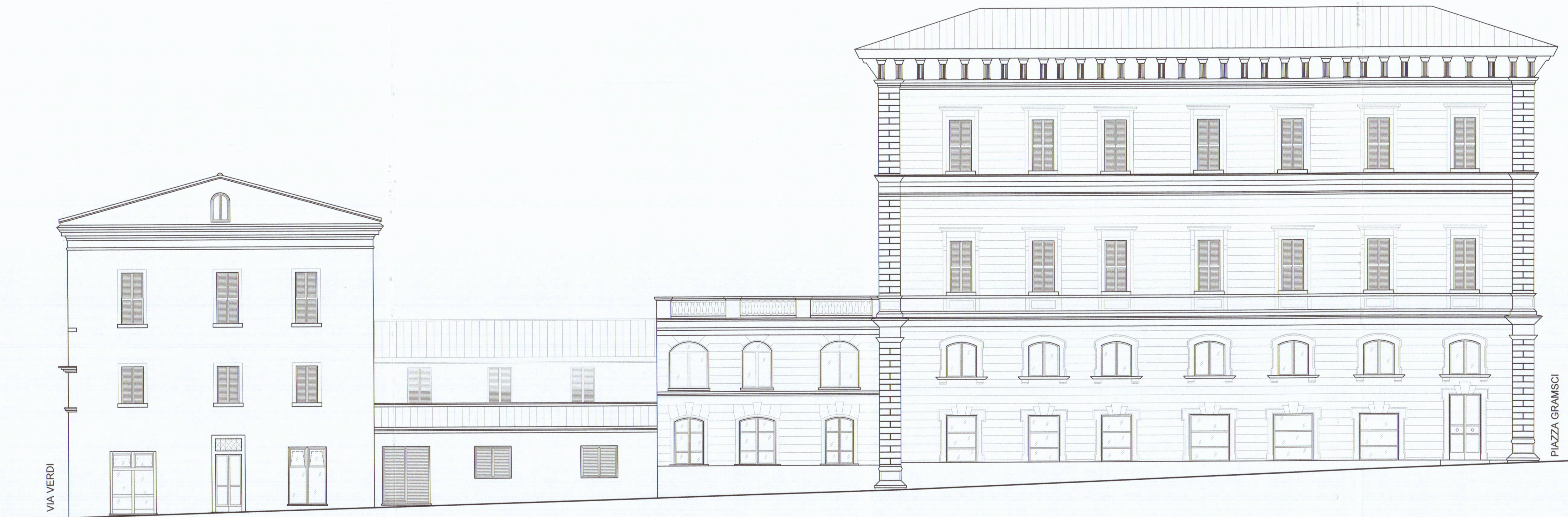
PROSPETTO SU VIA EUGENIO CHIESA
