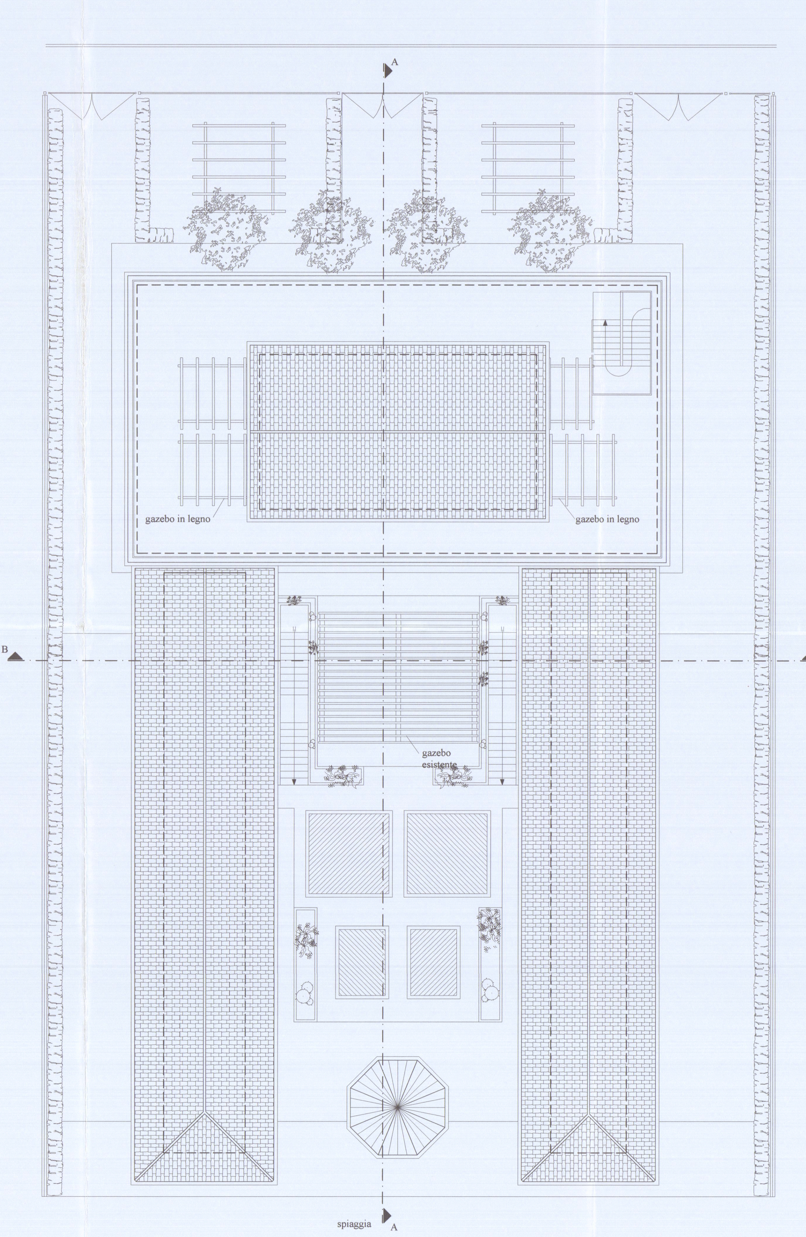
PIANTA COPERTURA
