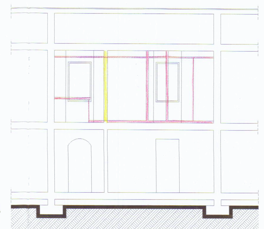
Sezione A - A (raffronto)
