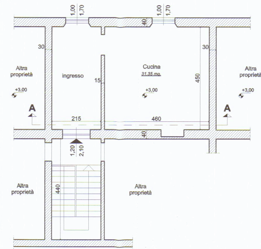
Piano Primo (Attuale)
