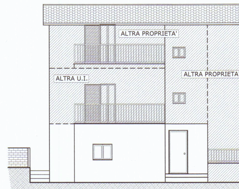
PROSPETTO OVEST
