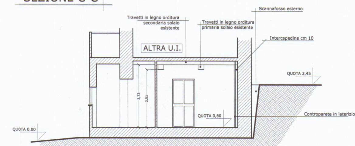
SEZIONE C-C'
