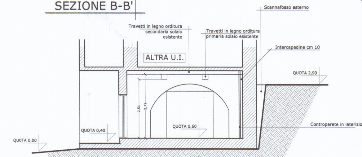
SEZIONE B-B'
