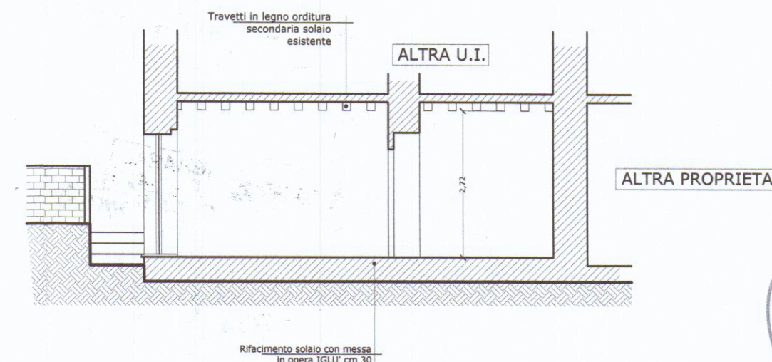
SEZIONE A-A'
