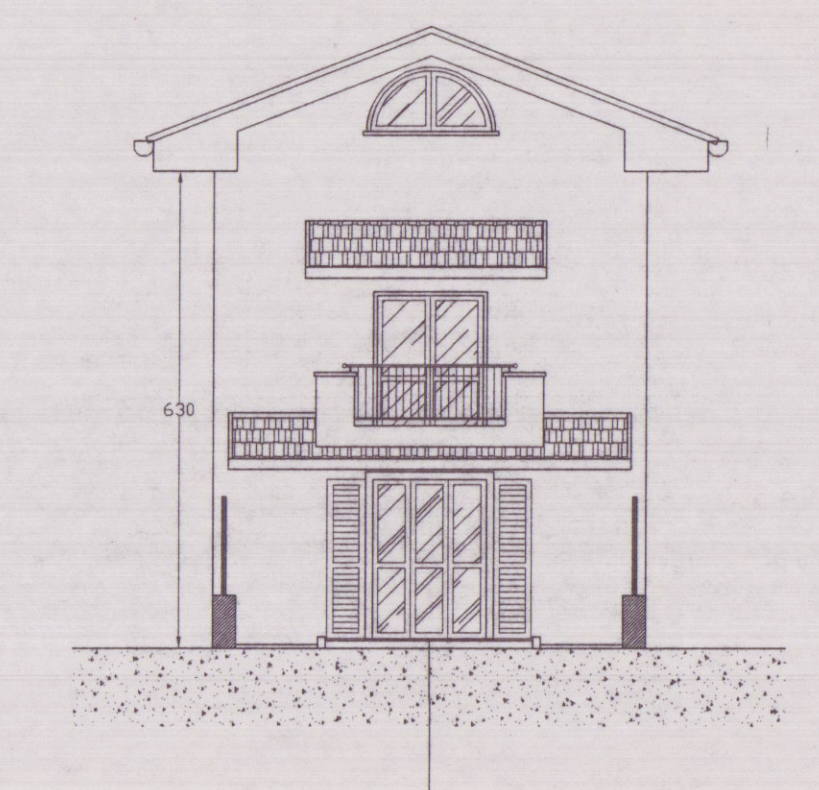
PROSPETTO SUD EST
