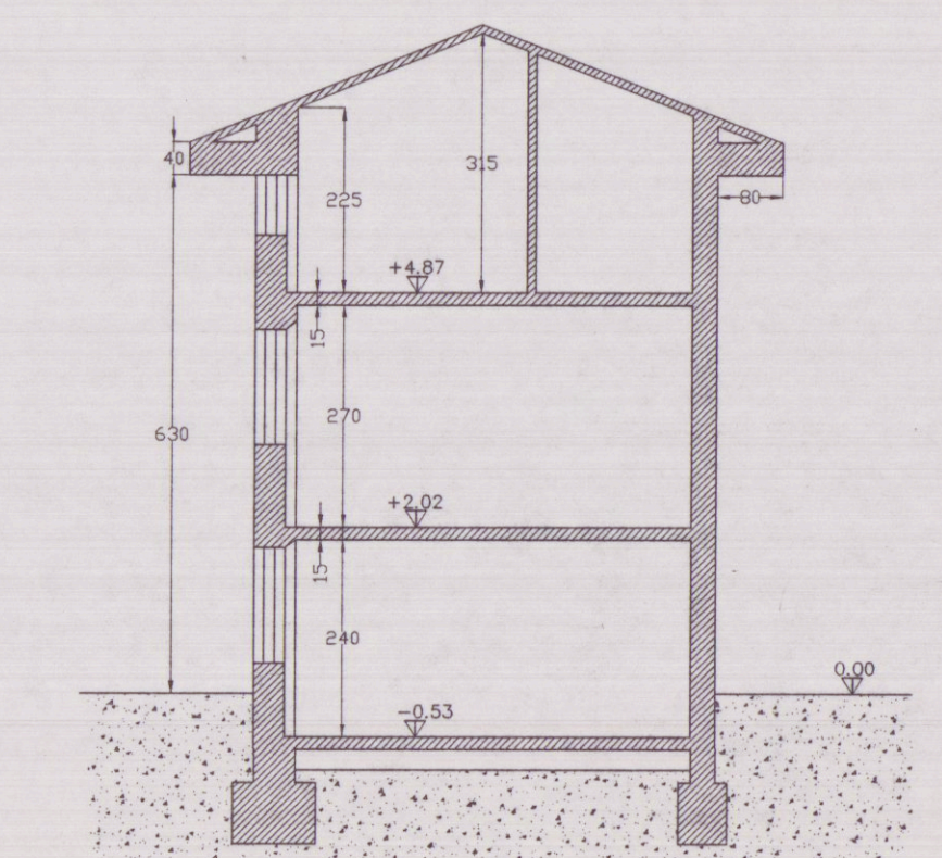
SEZIONE B-B
