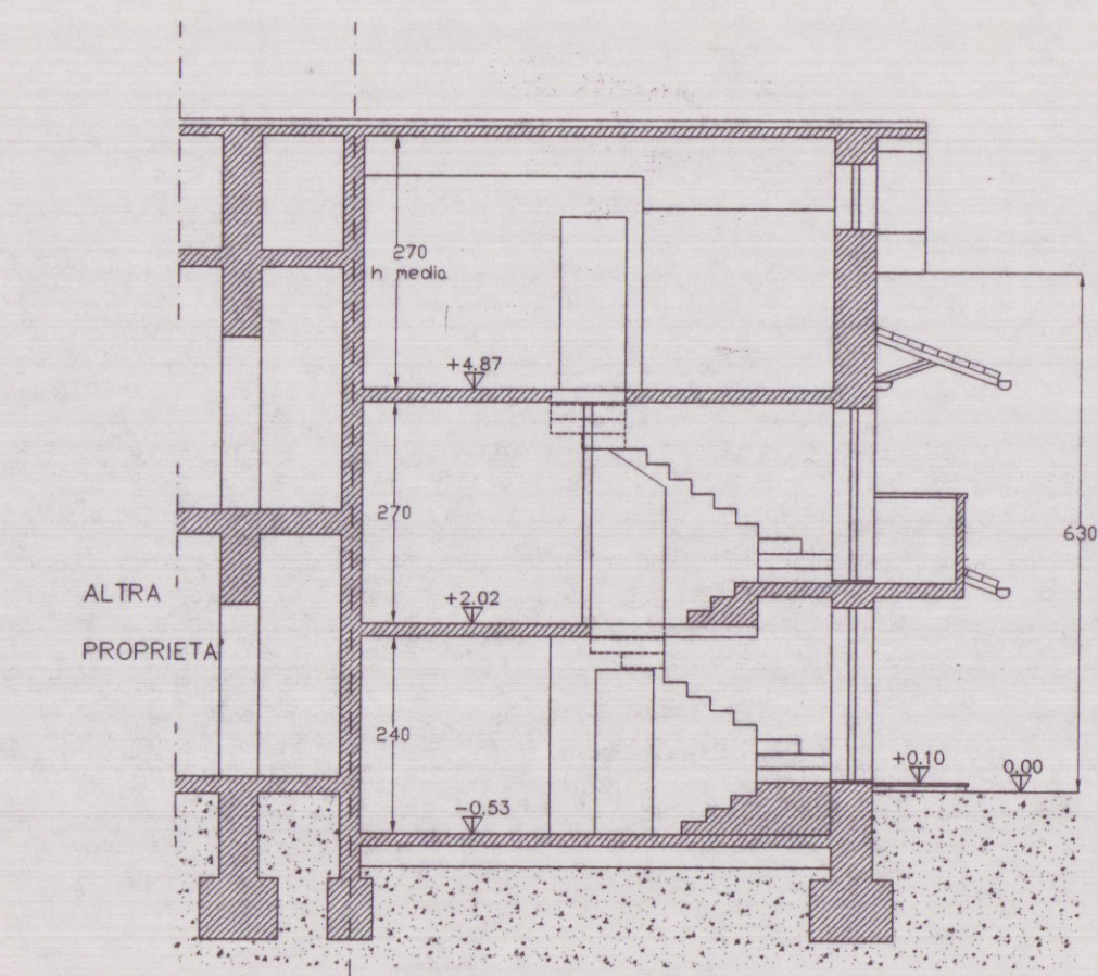
SEZIONE A-A
