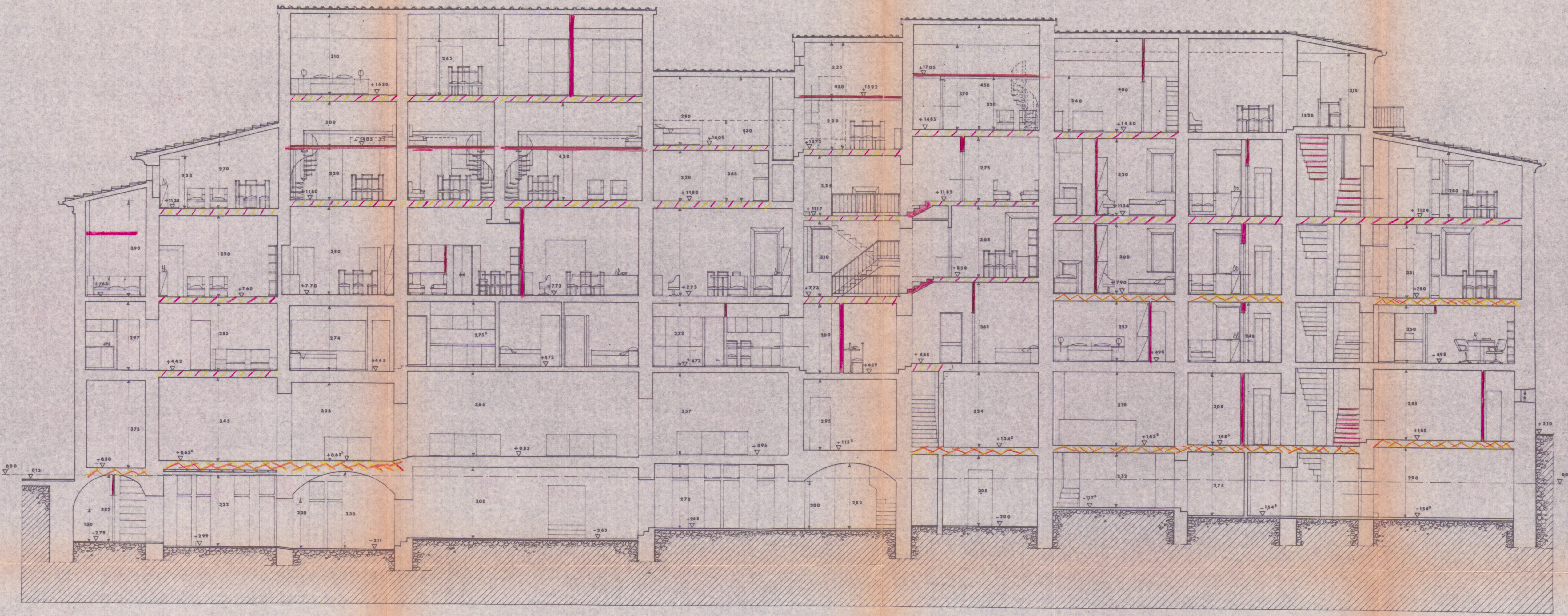
SEZIONE a-a
