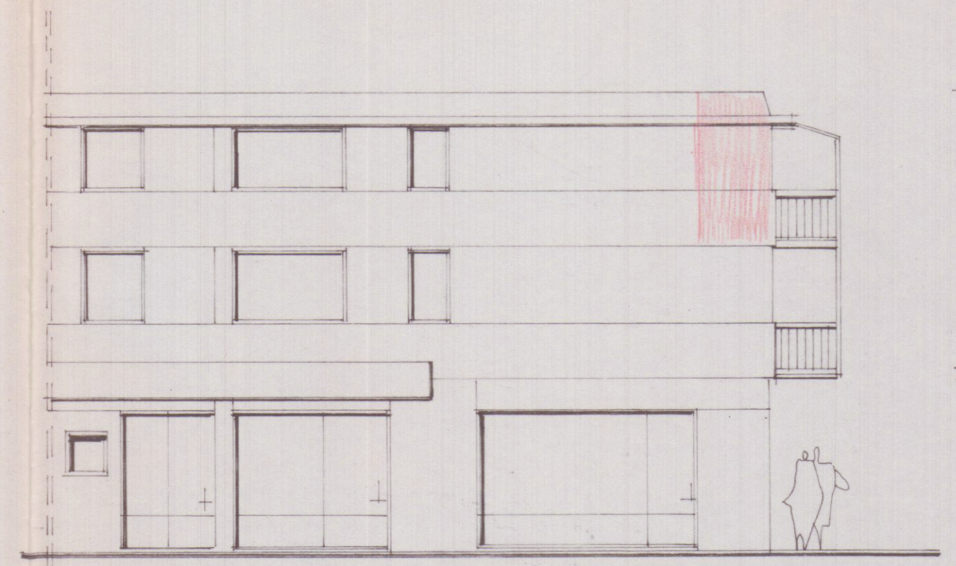
prospetto sud
