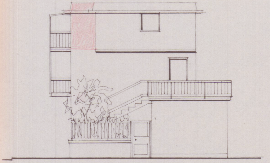
prospetto nord
