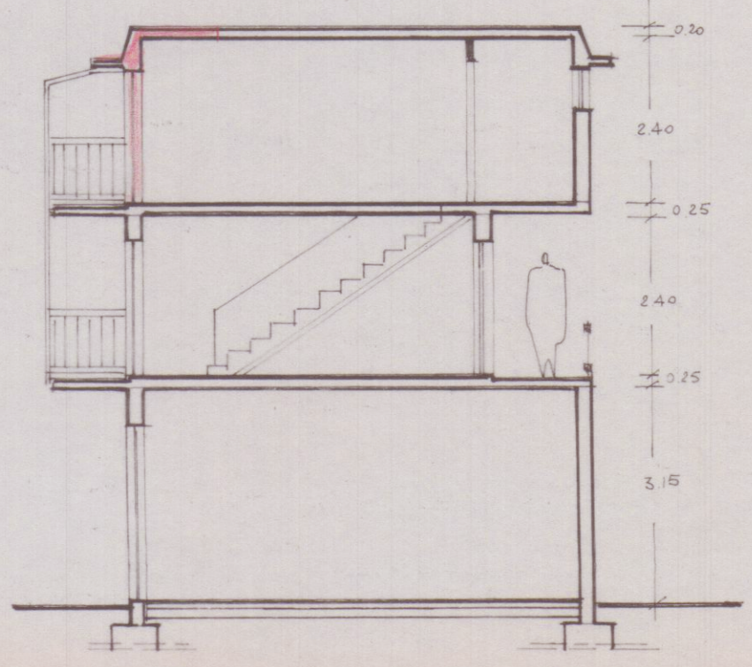
sezione
