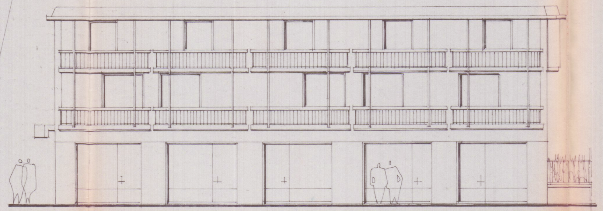
prospetto est
